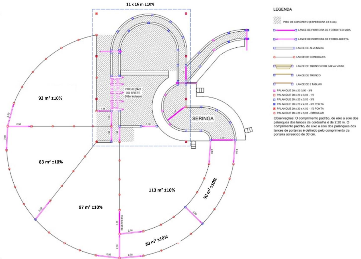
Figura 1. Desenho técnico de curral anti-stress para manejo de bovinos. (Área total construída: 620 m² ±10%).
