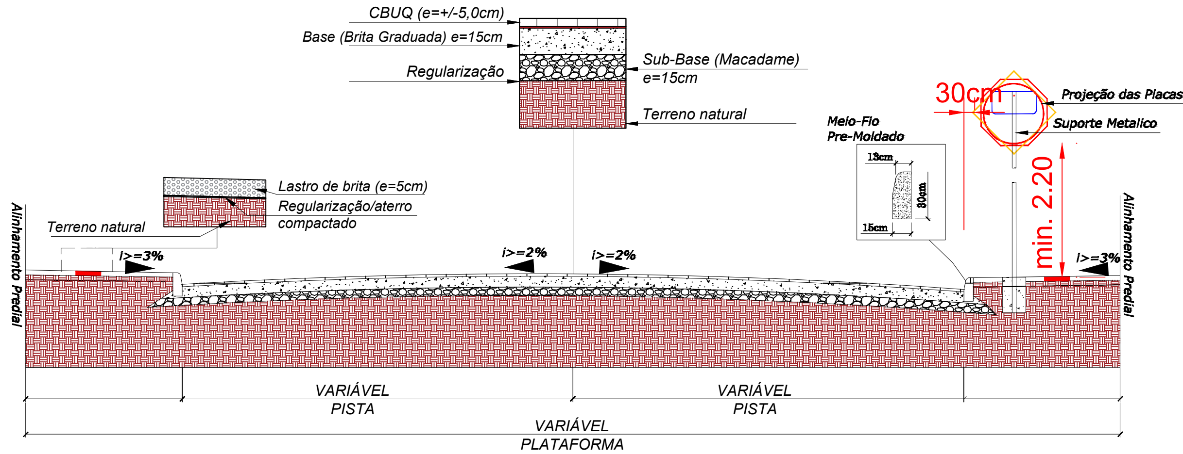
Seção Tipo - Geométrico, Pavimentação, Urbanísticos e Sinalização
