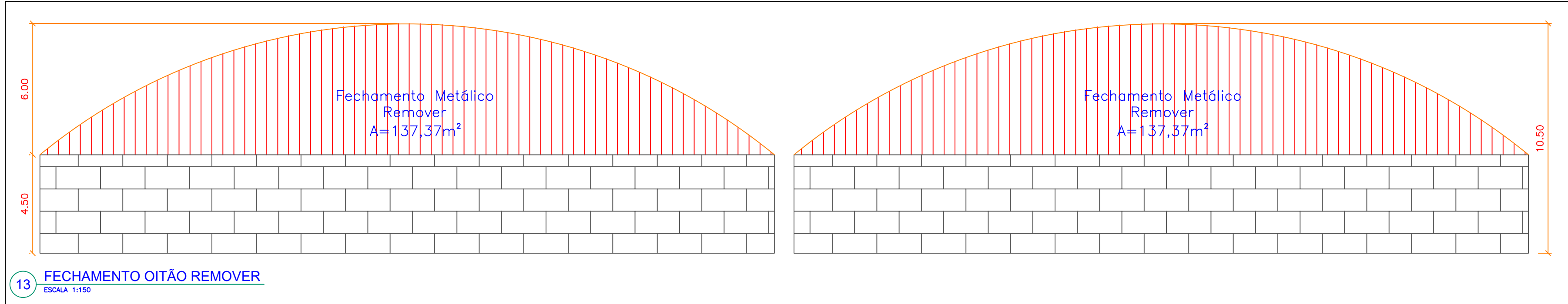
13 FECHAMENTO OITÃO REMOVER ESCALA 1:100
