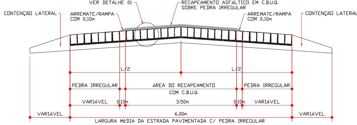
SEÇÃO TRANSVERSAL
