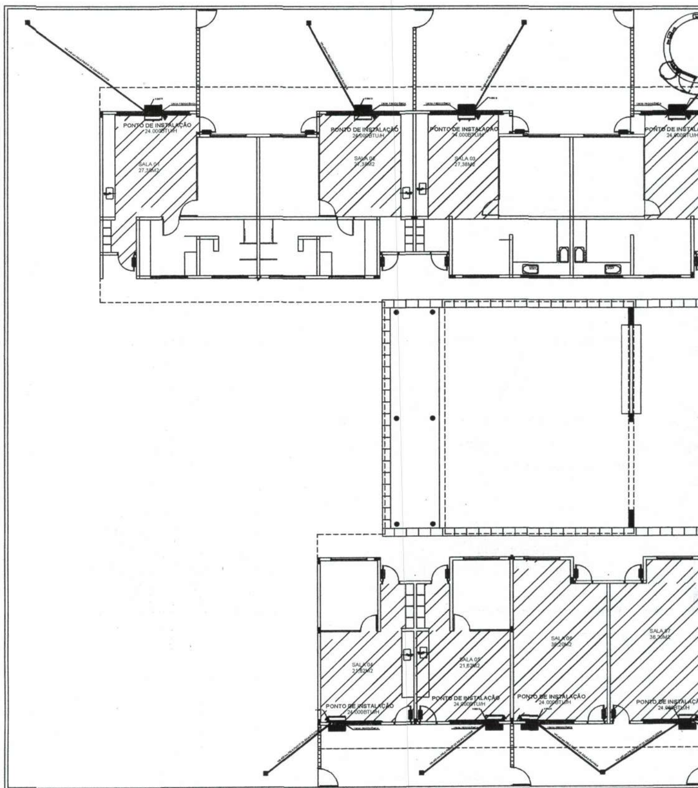
1 CROQUI INSTALAÇÃO AR CONDICIONADO - CMEI CLAUDIA HELENA NEGRAO S7 ESCALA
