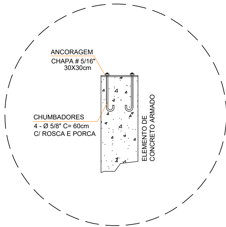
DETALHE TÍPICO DE FIXAÇÃO - CORTE S/ESCALA
