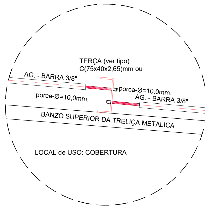
DET. AGULHAMENTO COB. S/ESCALA
