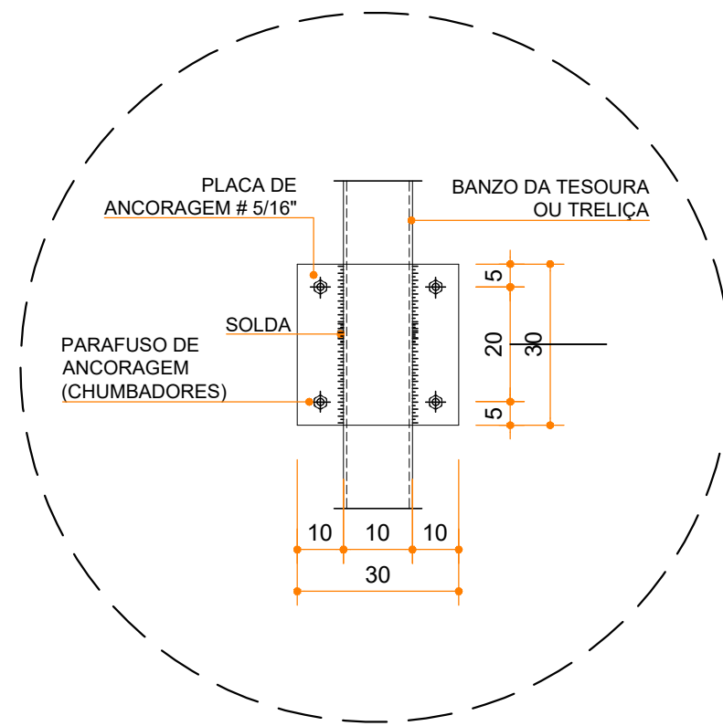
DETALHE TÍPICO DE FIXAÇÃO - PLANTA S/ESCALA
