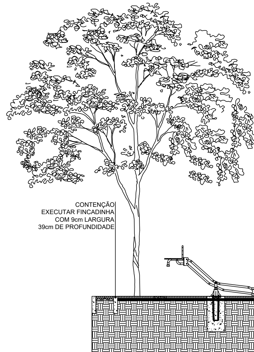
API 03 - CORTE AA' esc.:1:50
