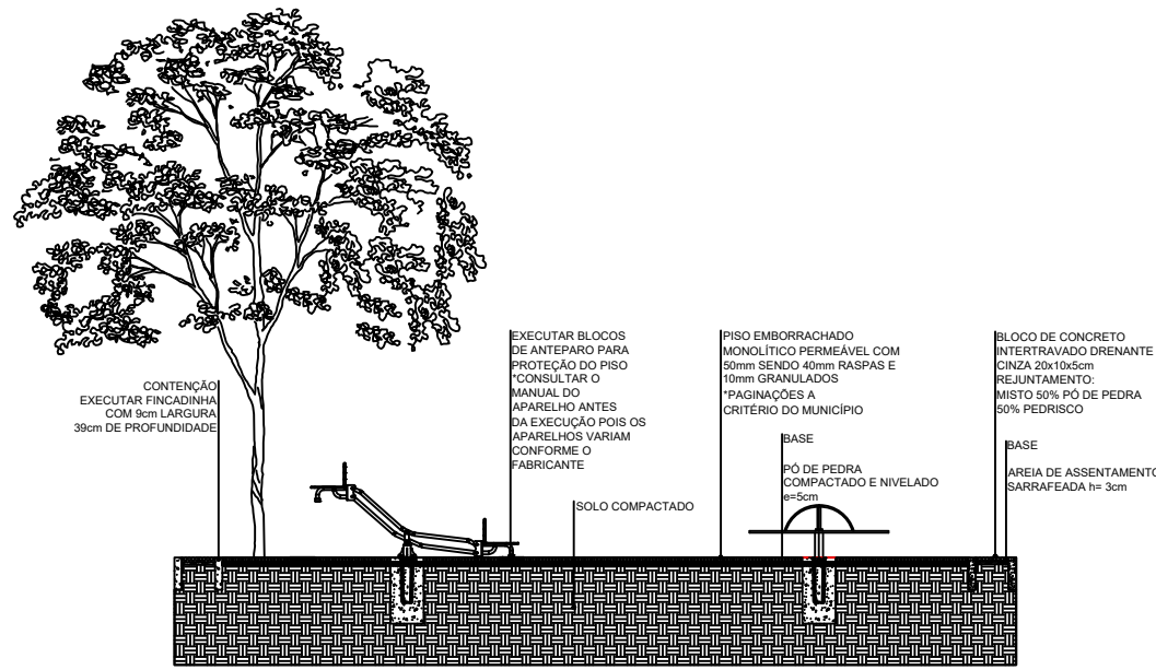
API 03 - CERCADO - CORTE AA' esc.:1:100
