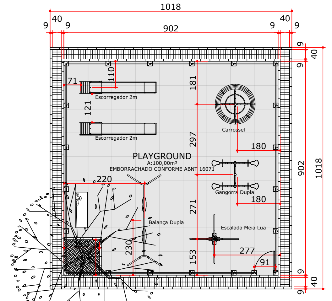
API 03 COM CERCA - PLANTA BAIXA esc.:1:100
