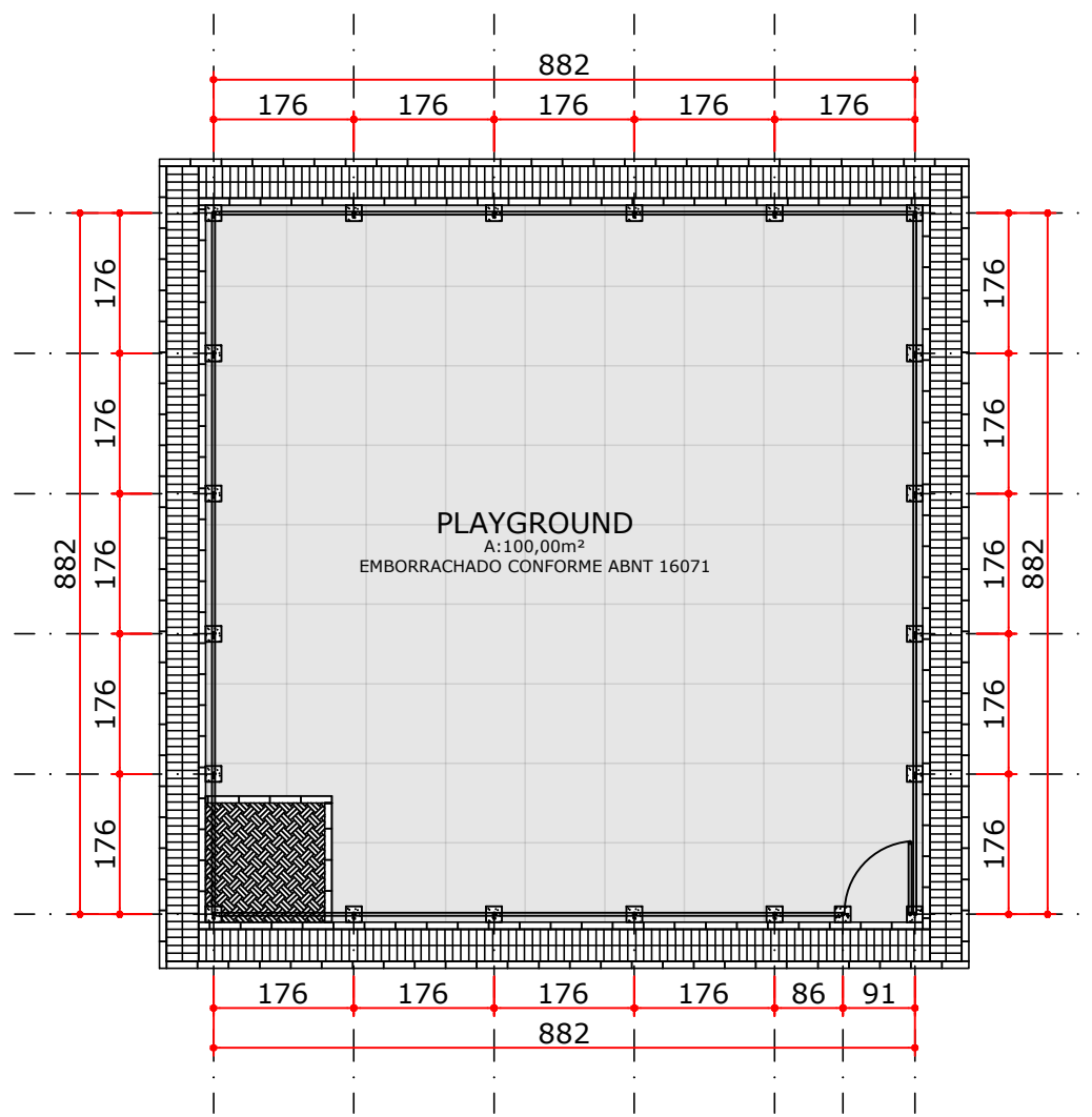
API 03 COM CERCA esc.:1:100
