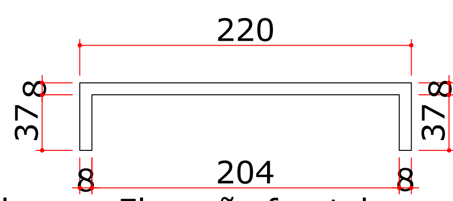
Elevação frontal
