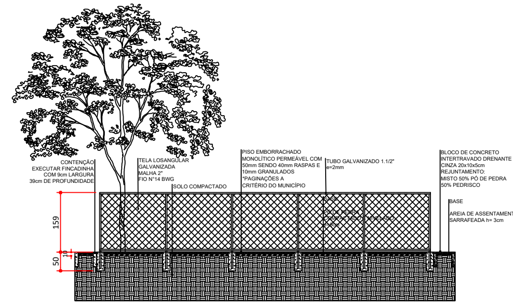
API 03 - GRADIL - CORTE AA' esc.:1:100
