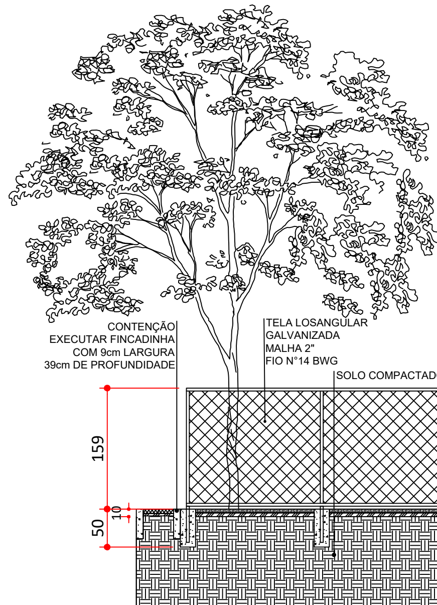
API 03 - GRADIL - CORTE AA' esc.:1:50
