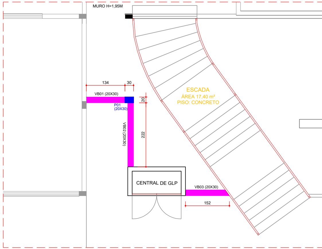
PLANTA BAIXA VIGA CINTA CENTRAL DE GLP ESC.: 1/75
