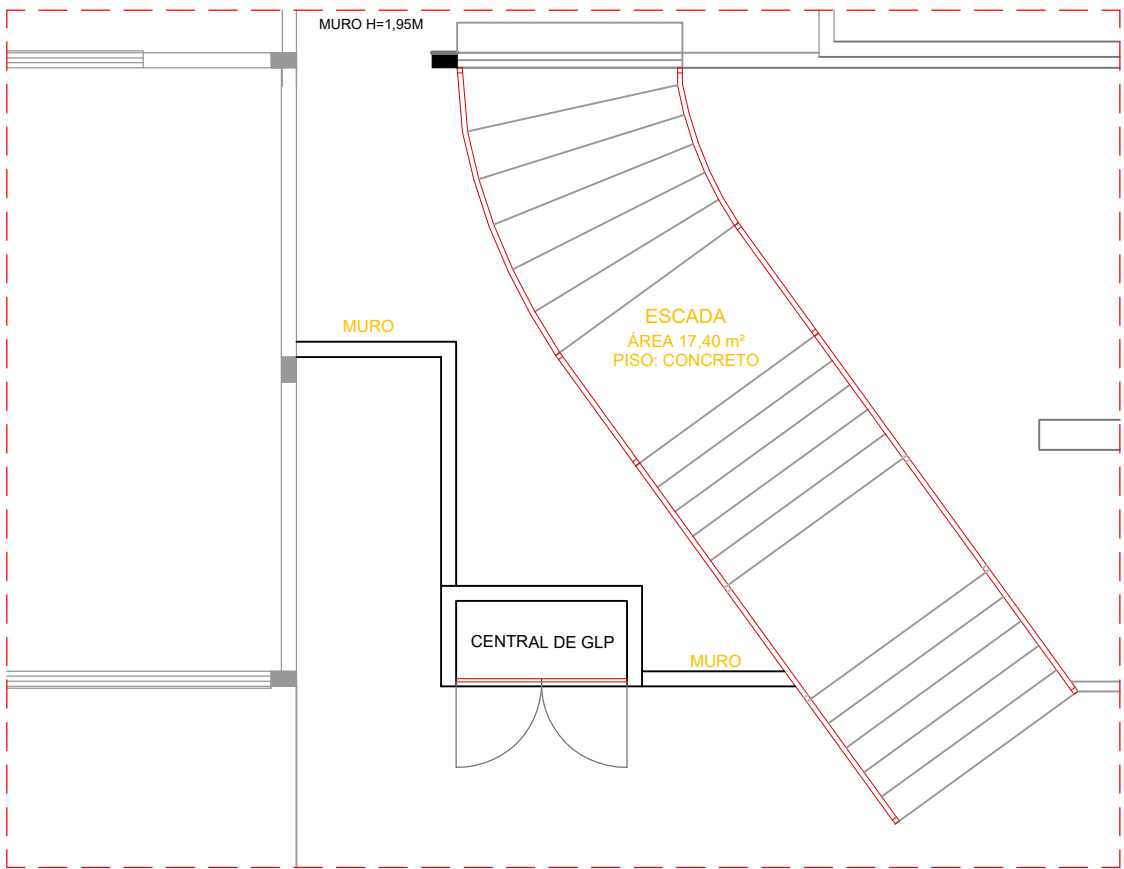
PLANTA BAIXA MURO CENTRAL DE GLP ESC.: 1/75
