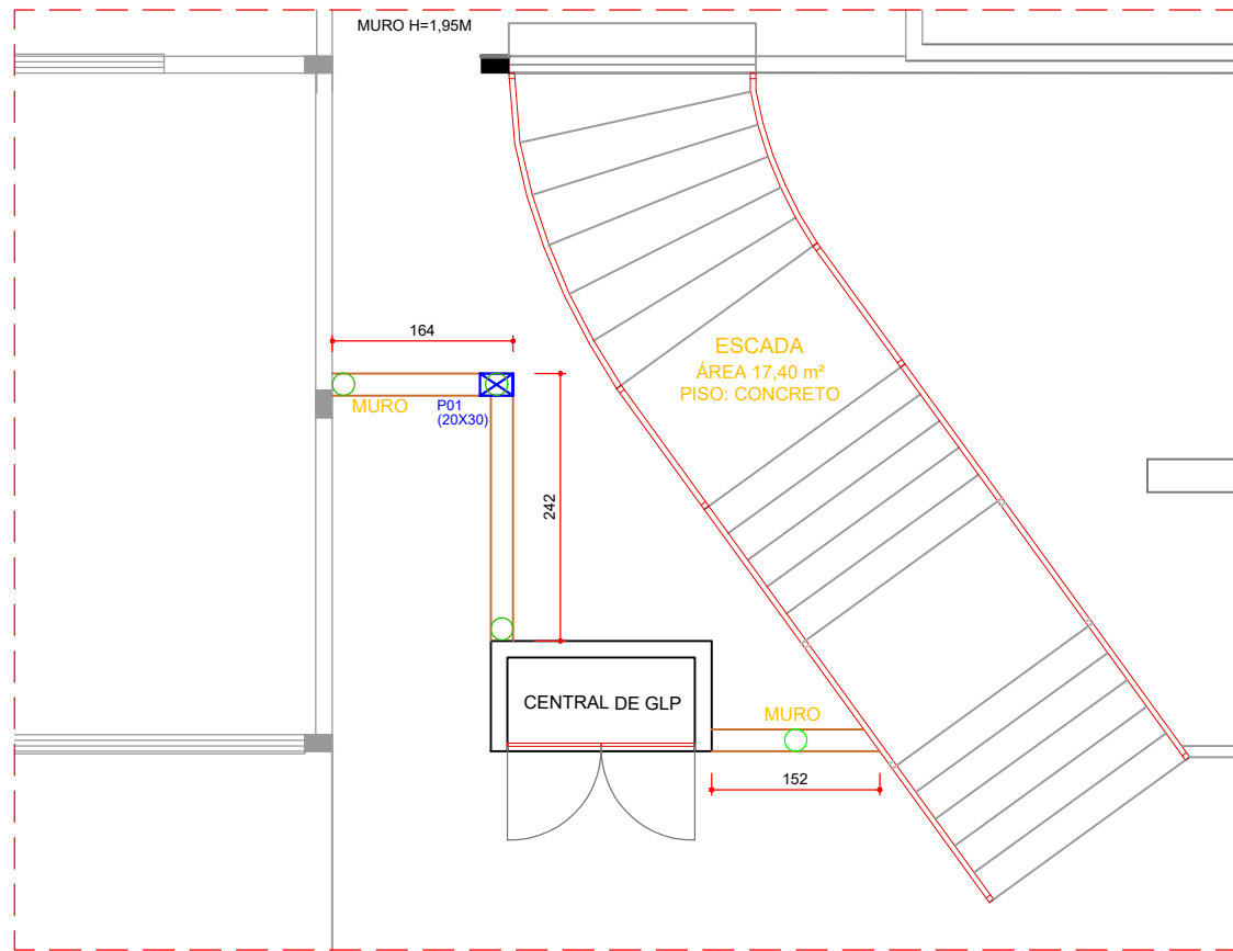
PLANTA BAIXA BALDRAME CENTRAL DE GLP ESC.: 1/75
