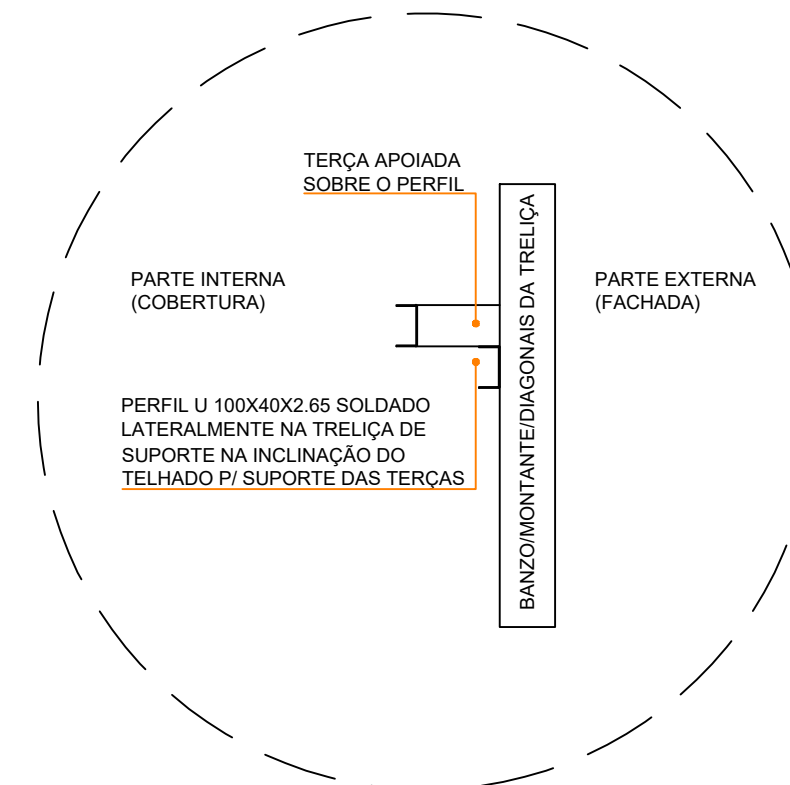
DETALHE 3 - FIXAÇÃO DE TERÇA EM TRELIÇA DE FACHADA S/ESCALA
