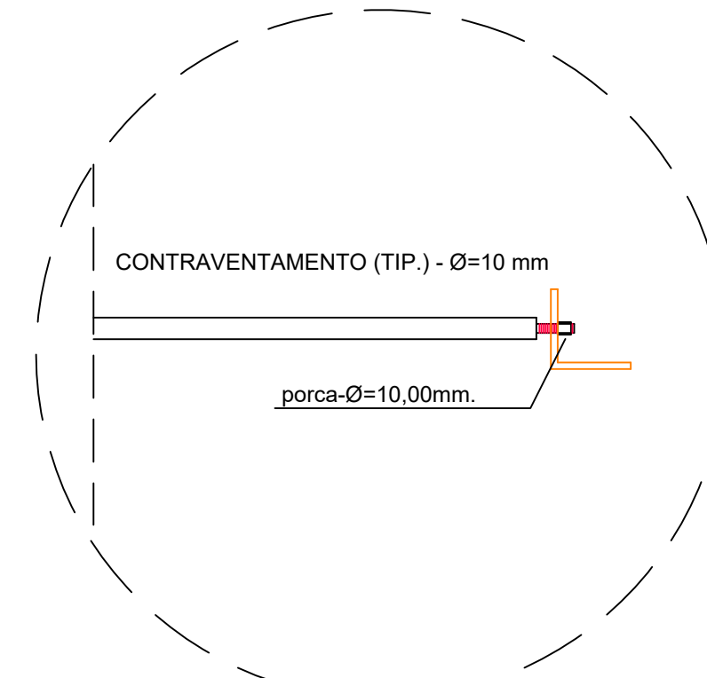
DETALHE DO CONTRAVENTAMENTO (TIP.) S/ESCALA
