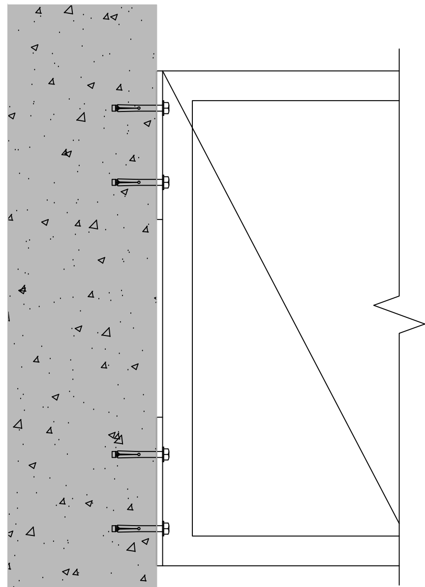
DETALHE DE FIXAÇÃO DAS TESOURAS/ TRELIÇAS EM BALANÇO ESCALA 1:5
