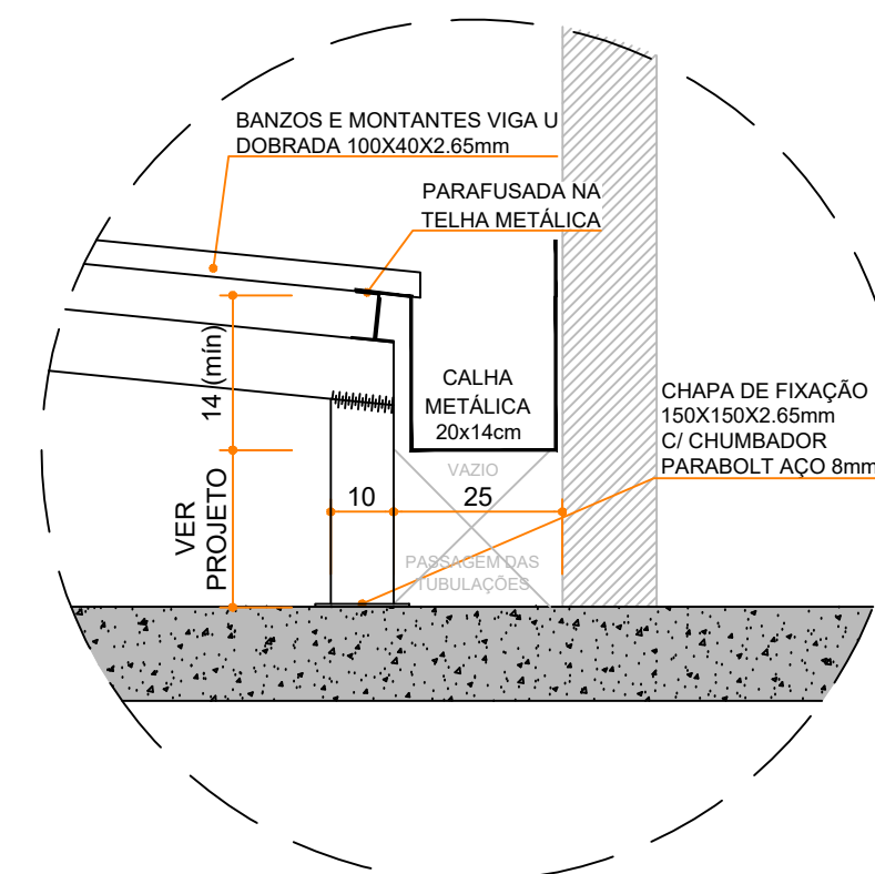
DETALHE DE FIXAÇÃO DA CALHA S/ESCALA
