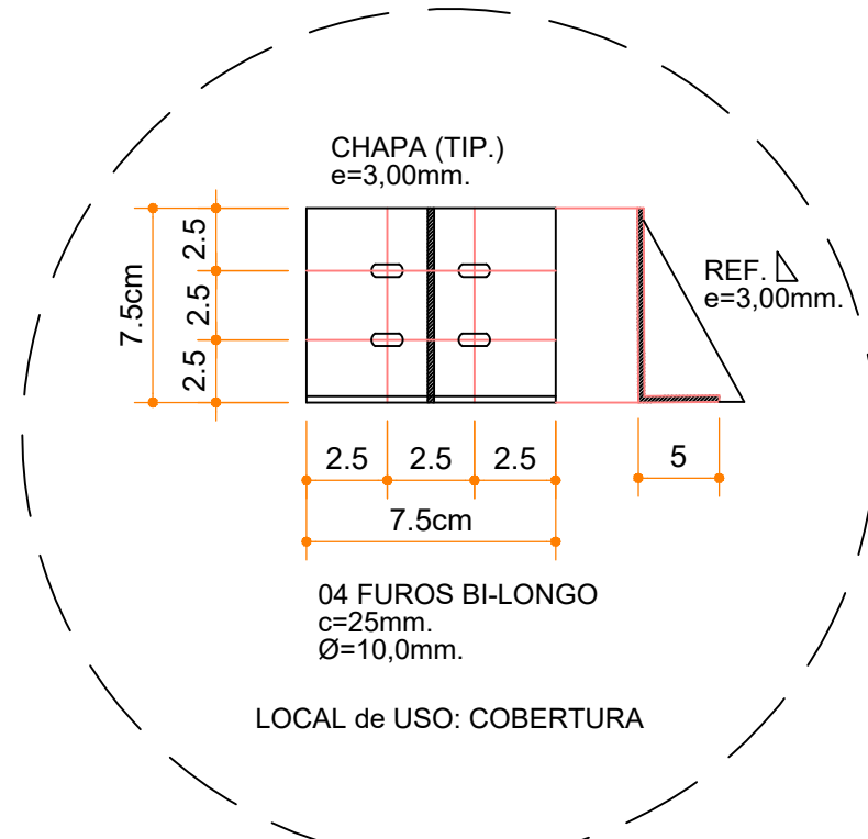
DET. FIXAÇÃO do TERÇAMENTO da COB. S/ESCALA
