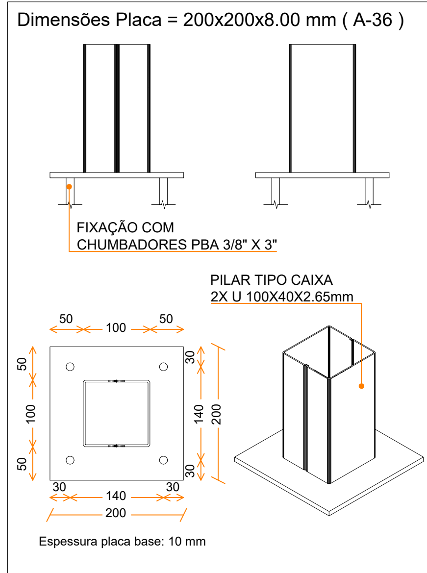
DETALHE DE FIXAÇÃO DO APOIO NA LAJE DE CONCRETO S/ESCALA
