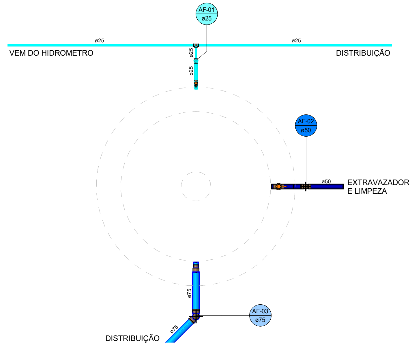
2 ÁGUA FRIA - CAIXA D'ÁGUA 1 : 25
