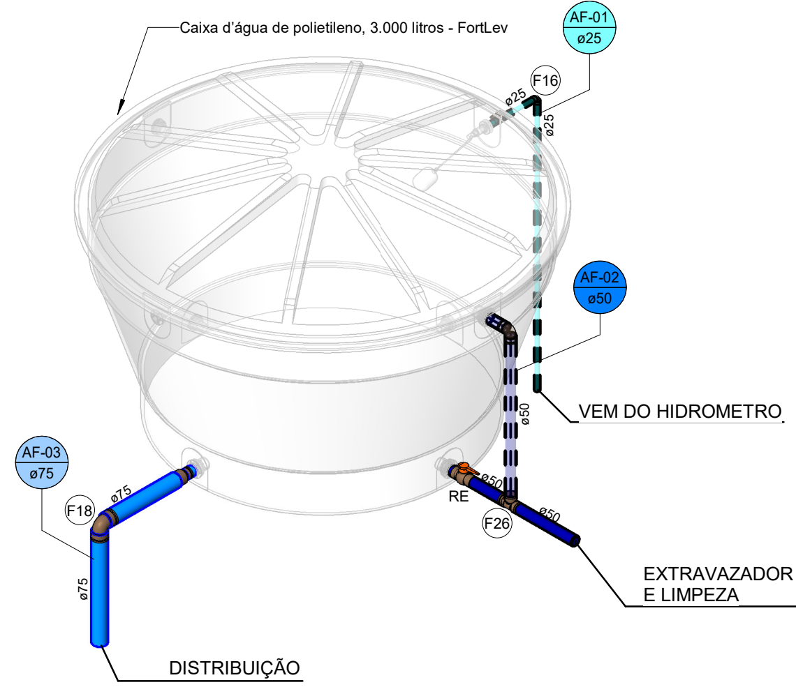
3 ISOMÉTRICO - CAIXA D'ÁGUA
