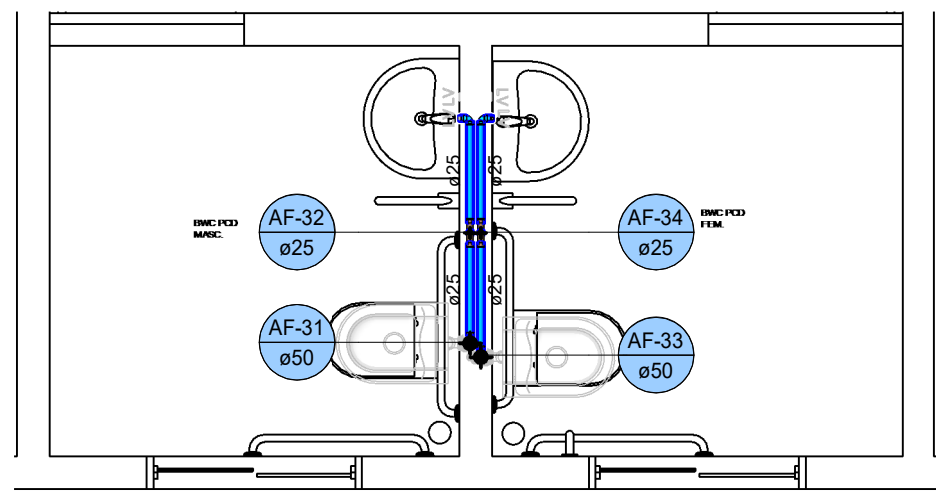
4 ÁGUA FRIA - BWC PCD MASC./PCD FEM. 1 : 35
