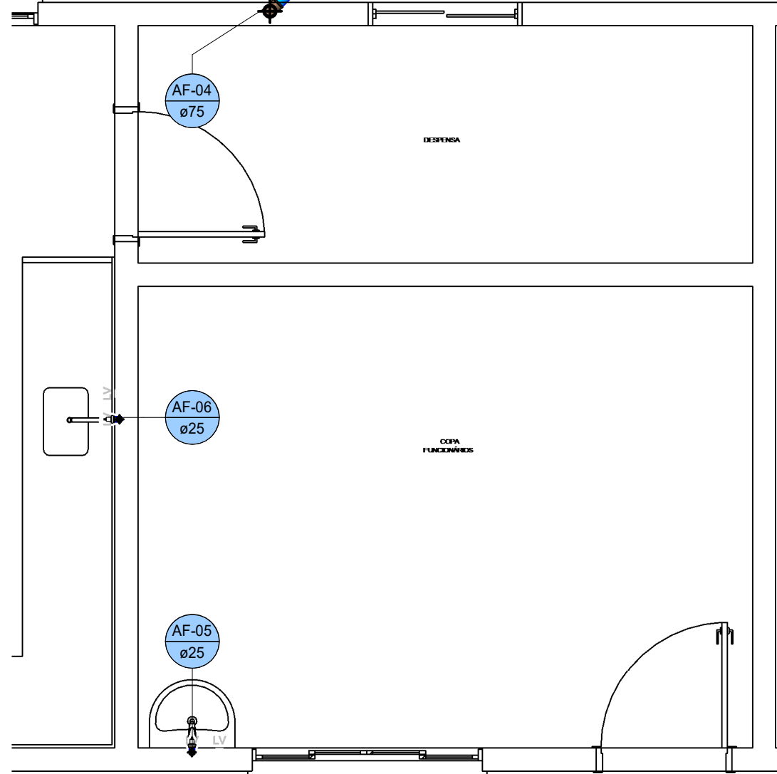
8 ÁGUA FRIA - COPA FUNC. 1 : 35
