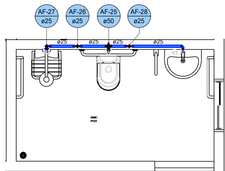
5 ÁGUA FRIA - BWC PCD. 1 : 35
