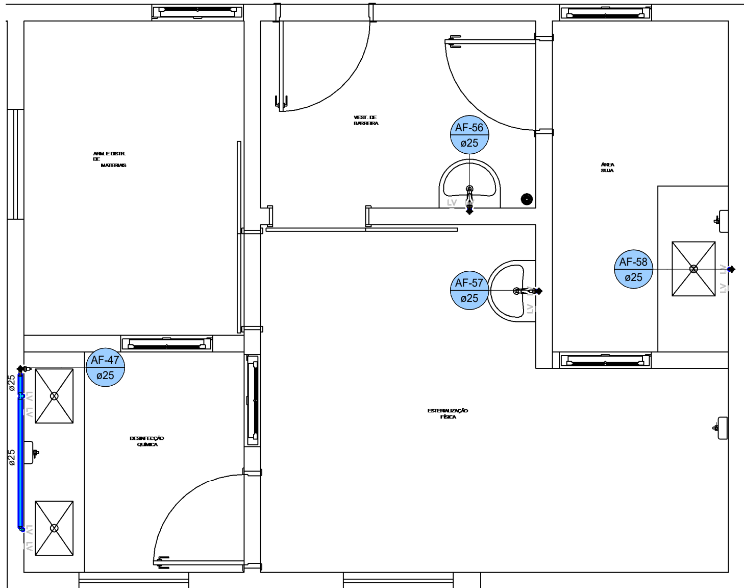
9 ÁGUA FRIA - ESTERILIZ. FÍSICA/Á. SUJA./VEST. DE BARR./DESINF. QUÍMICA 1 : 35
