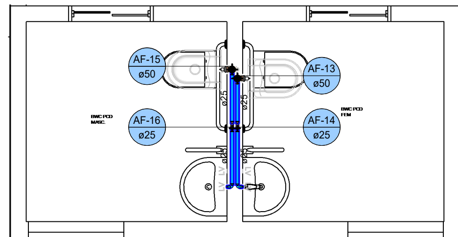
3 ÁGUA FRIA - BWC PCD MASC./FEM. 1 : 35
