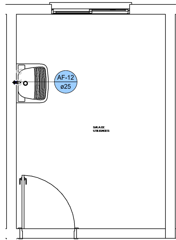
13 ÁGUA FRIA - SALA DE UTILIDADES 1 : 35
