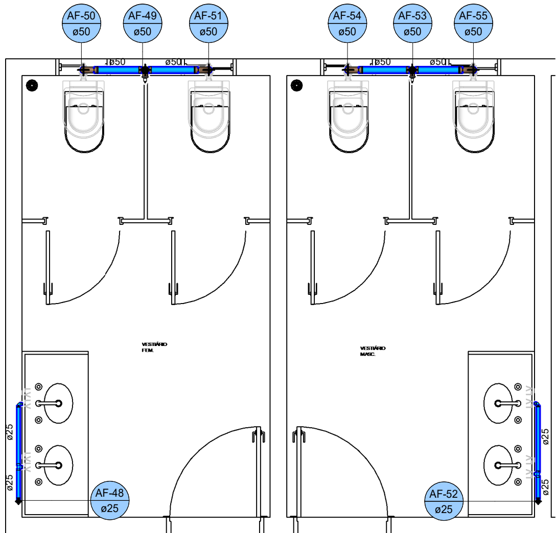
14 ÁGUA FRIA - VEST. FEM./MASC. 1 : 35
