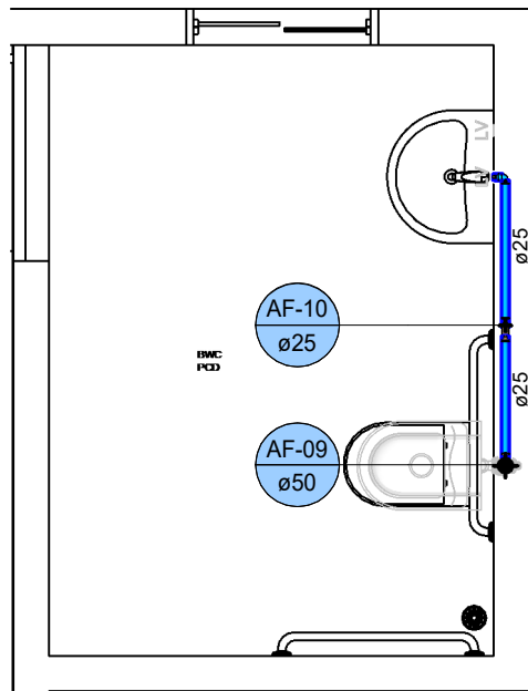
1 ÁGUA FRIA - BWC PCD 1 : 35
