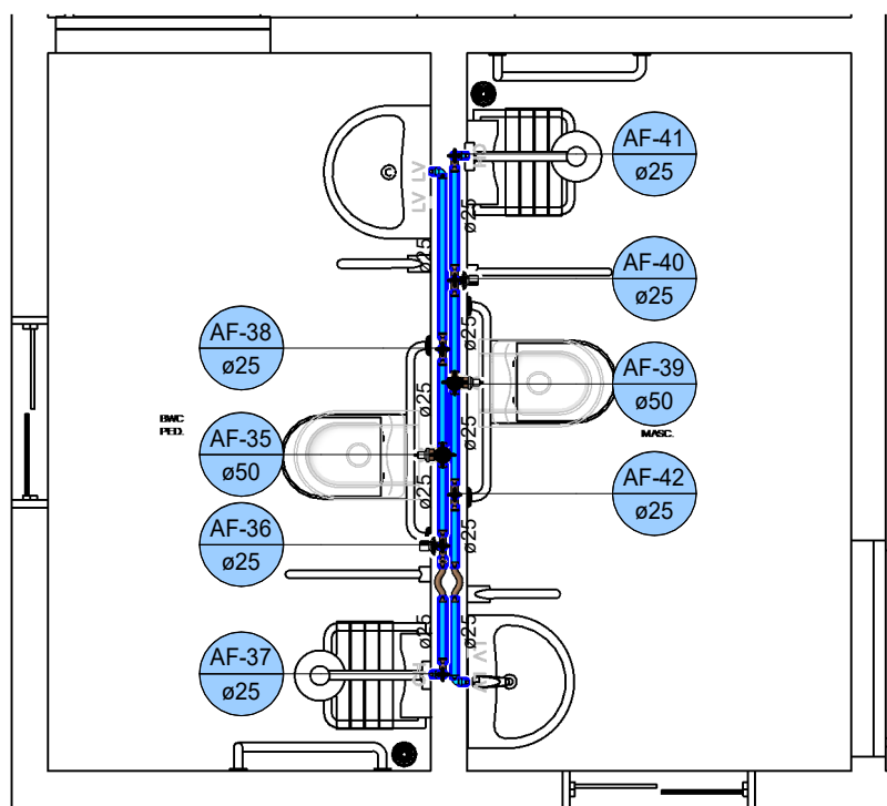
6 ÁGUA FRIA - BWC PED./MASC. 1 : 35
