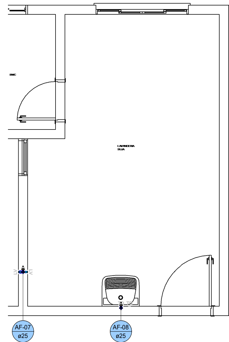
15 ÁGUA FRIA - LAVAND. SUJA 1 : 35
