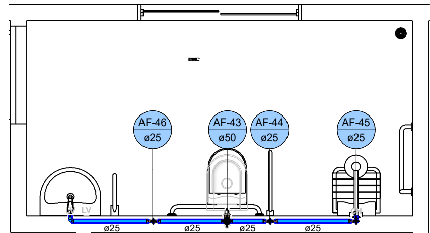
2 ÁGUA FRIA - BWC 1 : 35
