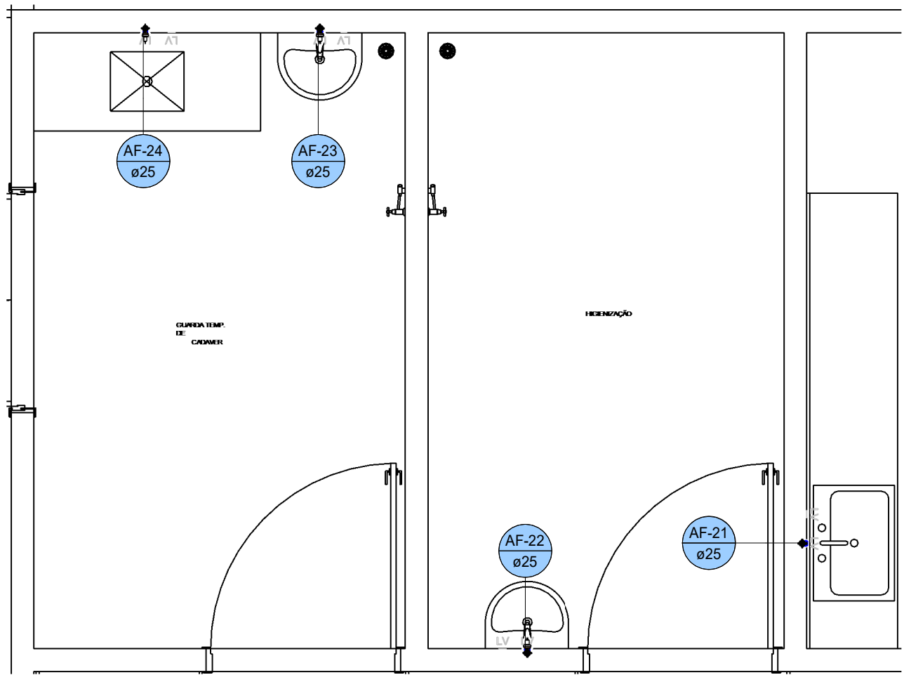
10 ÁGUA FRIA - GUARDA TEMP. DE CADAVER/HIGIENIZAÇÃO 1 : 35
