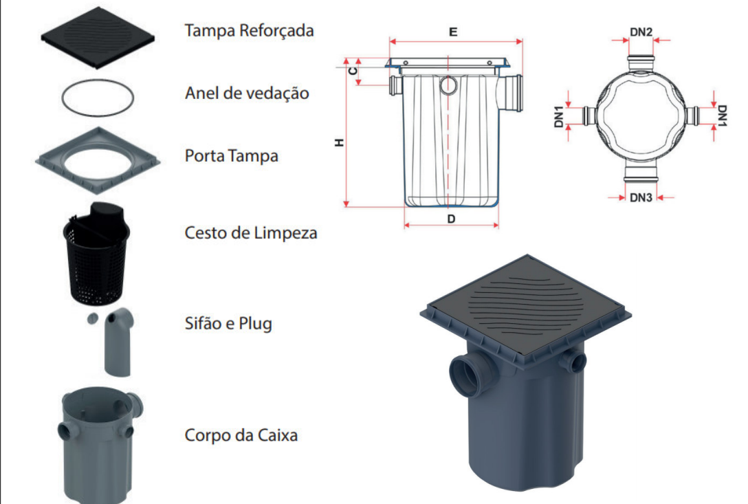
Detalhes - Caixa de Gordura Pequena (CGP) - 18 Litros - TIGRE
