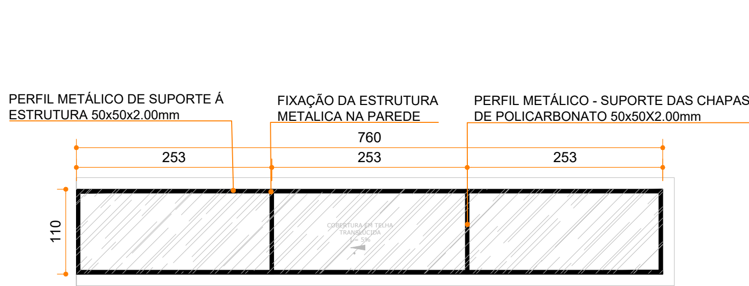
COBERTURA EM TELHA TRANSLÚCIDA 01 ESCALA: 1/50
