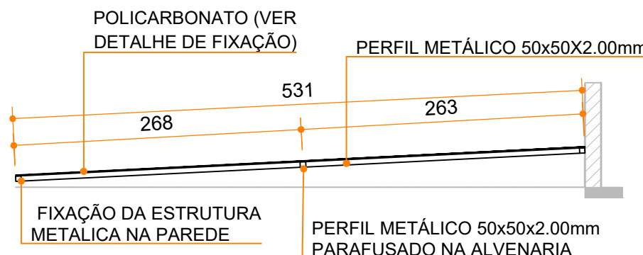
CORTE ESCALA: 1/50
