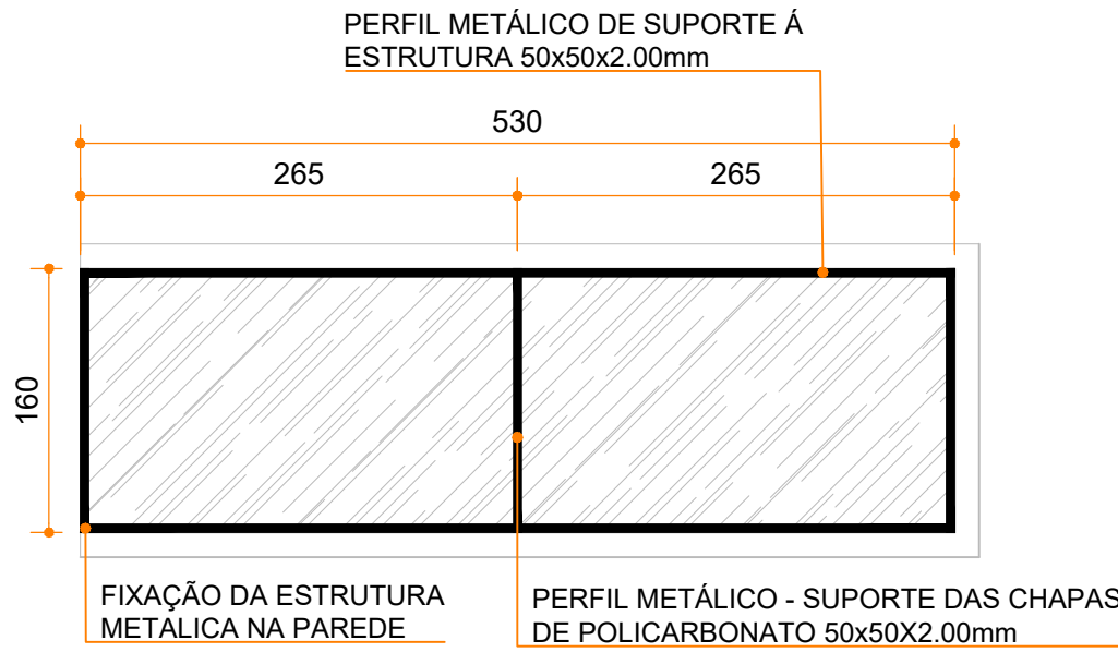
COBERTURA EM TELHA TRANSLÚCIDA 02 ESCALA: 1/50
