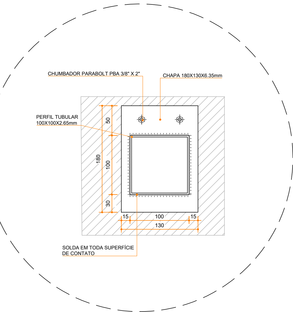
DETALHE DE FIXAÇÃO COBERTURA METÁLICA SEM ESCALA
