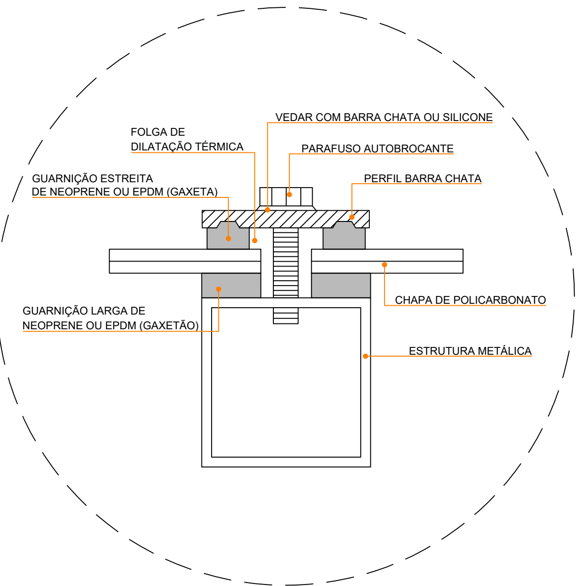
DETALHE DE FIXAÇÃO DAS CHAPAS DE POLICARBONATO SEM ESCALA
