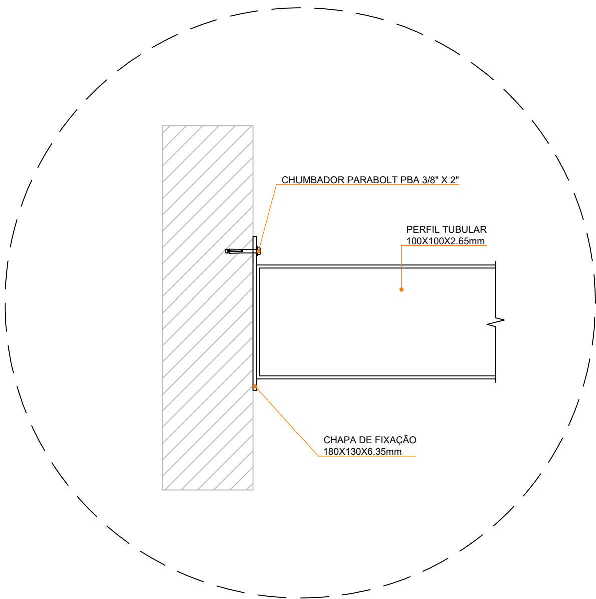
DETALHE DE FIXAÇÃO COBERTURA METÁLICA SEM ESCALA
