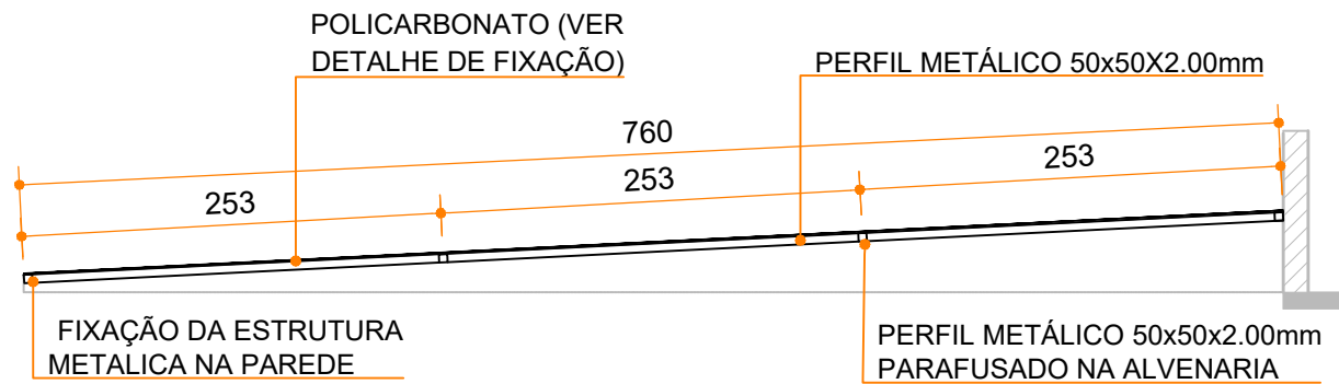
CORTE ESCALA: 1/50
