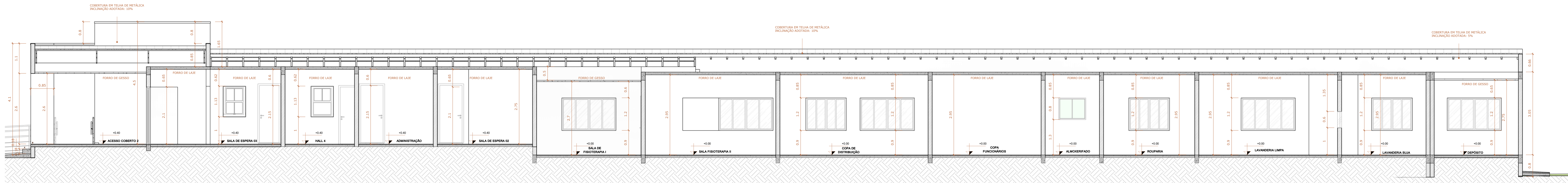
CORTE AA ESCALA 1:50
