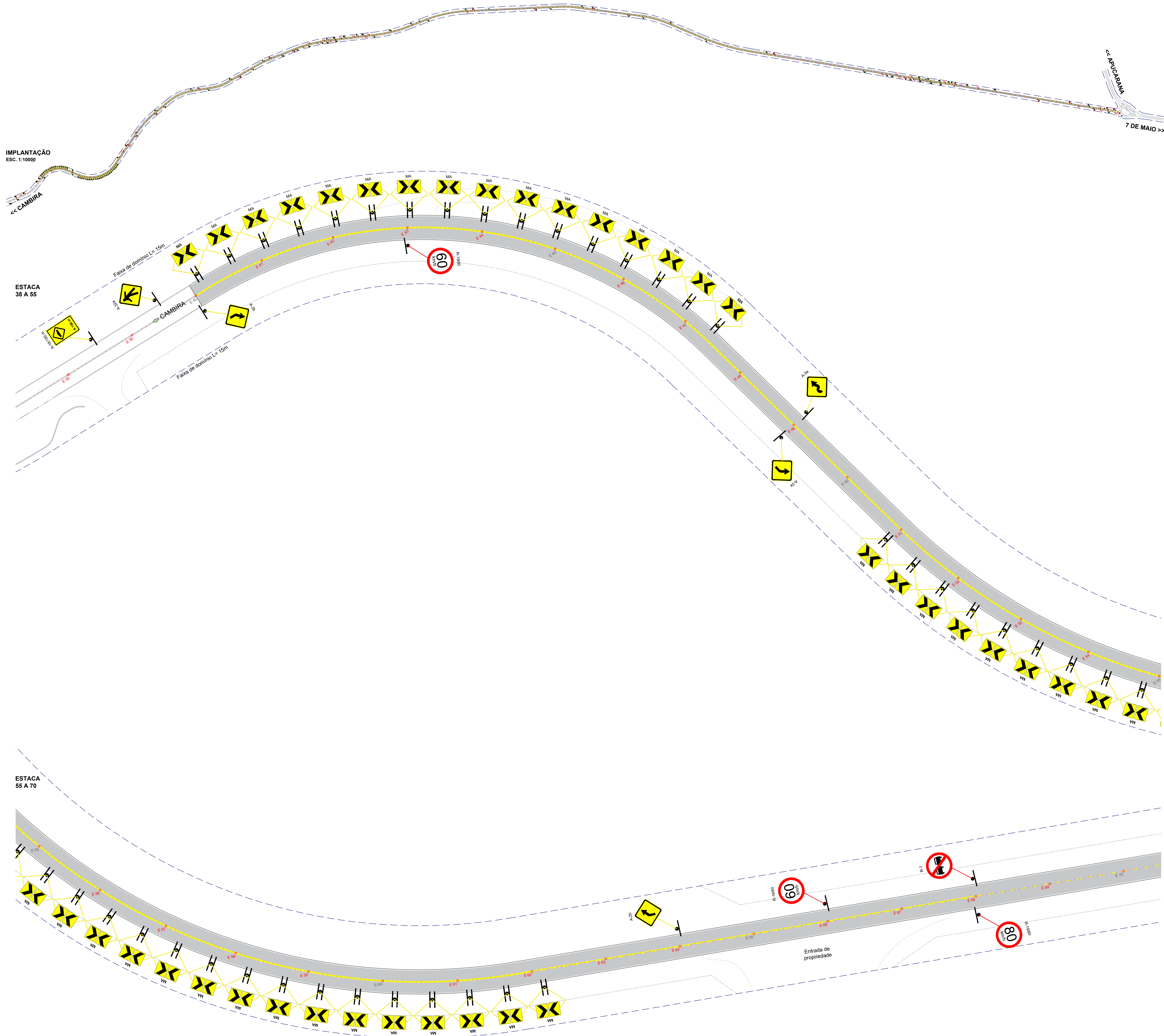
MARCADORES DE ALINHAMENTO - MA SEM ESCALA
