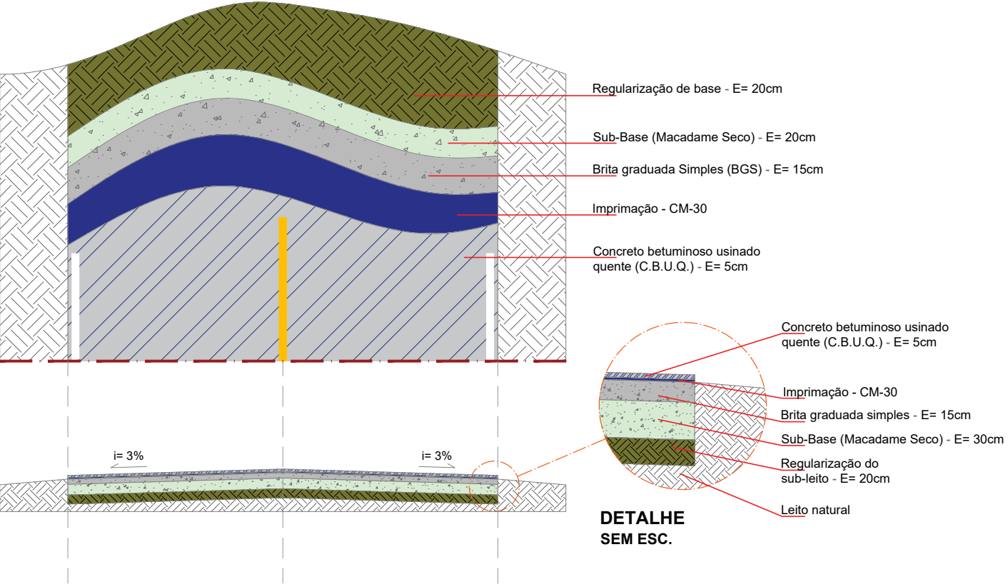
SECÇÃO TRANSVERSAL - DETALHAMENTO | ESTACA 00 a 551 SEM ESCALA
