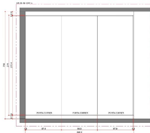
ELEVAÇÃO 01 - DETALHAMENTO ARMÁRIO 02
