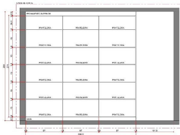
ELEVAÇÃO 01 - DETALHAMENTO ARMÁRIO 02 PARTE INTERNA
