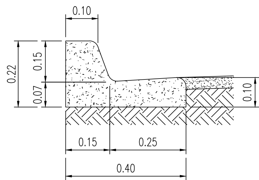
MEIO-FIO COM SARJETA
