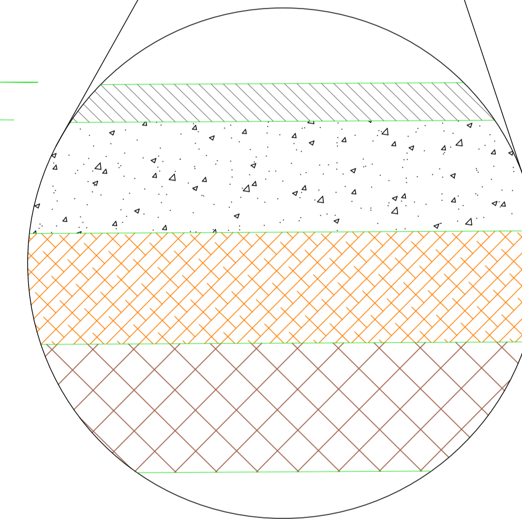
DETALHE DE PAVIMENTAÇÃO - DET.02 SEM ESCALA
