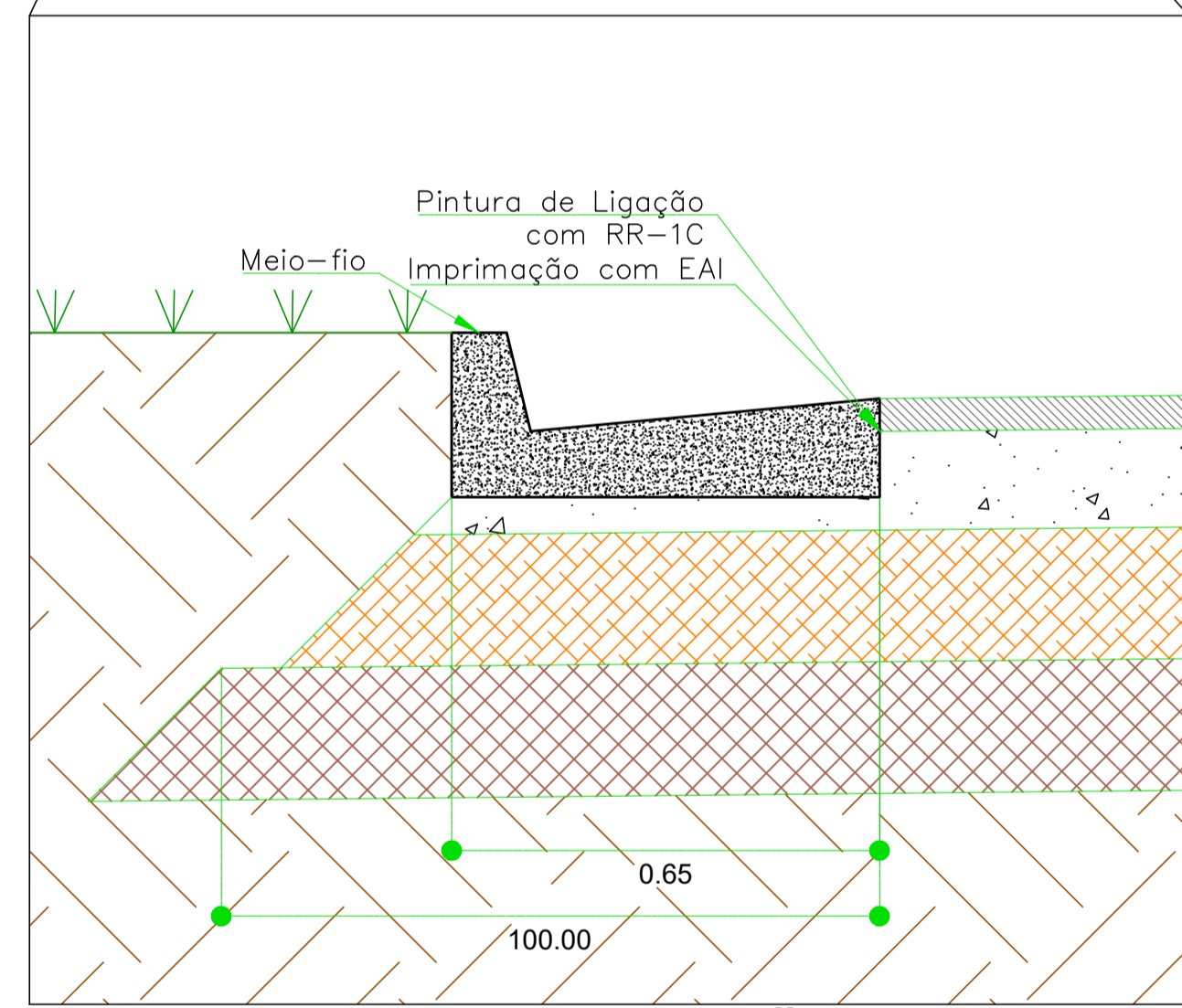
DETALHE DE PAVIMENTAÇÃO - DET.01 SEM ESCALA
