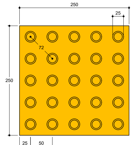
DETALHE "2" S/ ESC. DETALHE DO PISO TÁTIL DE ALERTA
