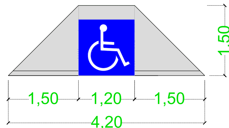
DETALHE "1" S/ ESC. RAMPA DE ACESSIBILIDADE
