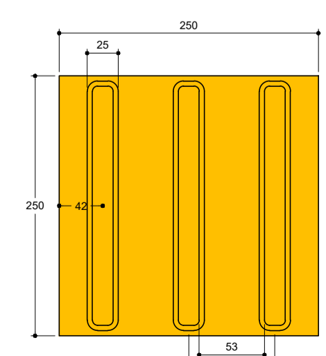
DETALHE "3" S/ ESC. DETALHE DO PISO TÁTIL DIRECIONAL
