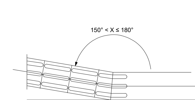
DETALHE "4" S/ ESC. MUDANÇA DE DIREÇÃO 150° < X ≤ 180°
