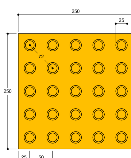
DETALHE "2" S/ ESC. DETALHE DO PISO TÁTIL DE ALERTA
