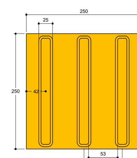
DETALHE "3" S/ ESC. DETALHE DO PISO TÁTIL DIRECIONAL
