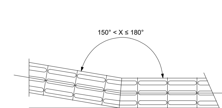
DETALHE "4" S/ ESC. MUDANÇA DE DIREÇÃO 150° < X ≤ 180°
