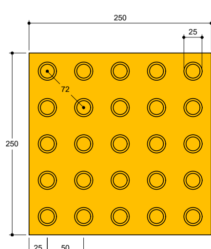
DETALHE "2" S/ ESC. DETALHE DO PISO TÁTIL DE ALERTA
