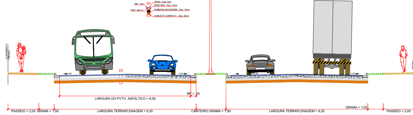
SEÇÃO TIPO - IMPLANTAÇÃO ESC: 1/500
