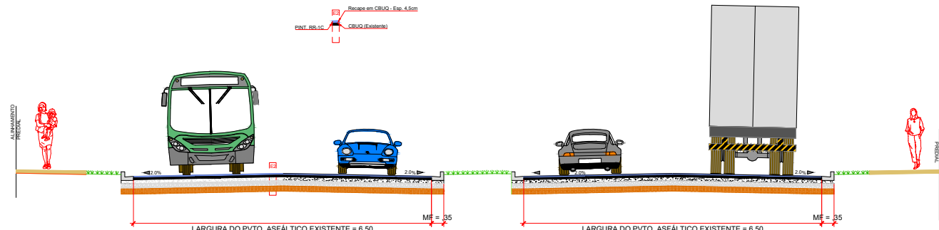
SEÇÃO TIPO - RECAPEAMENTO ESC: 1/500
