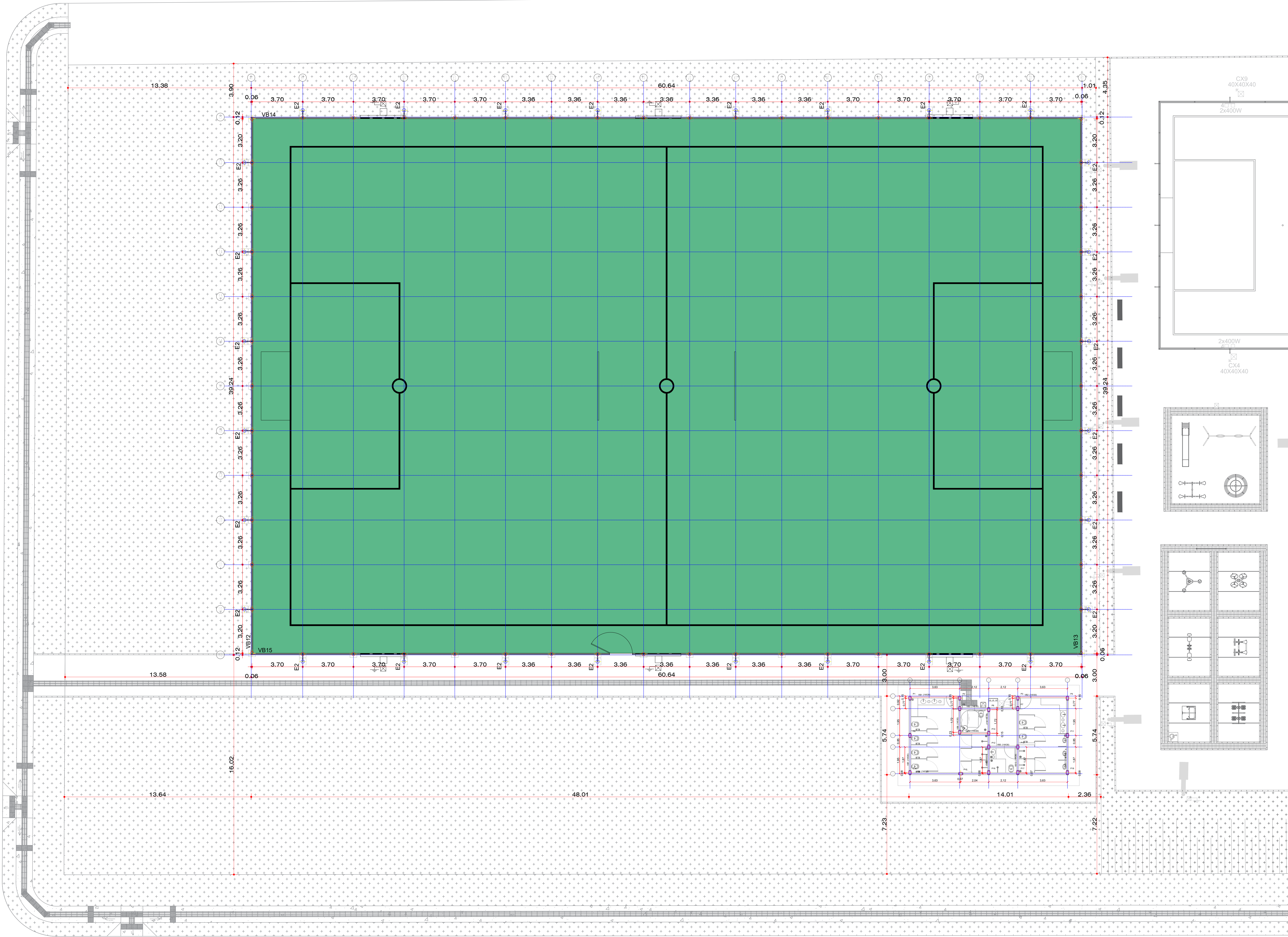
IMPLANTAÇÃO GERAL - LOCAÇÃO DE ESTACAS Escala 1:100
