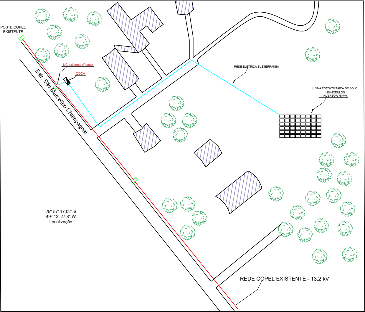
1 PLANTA DE SITUAÇÃO
