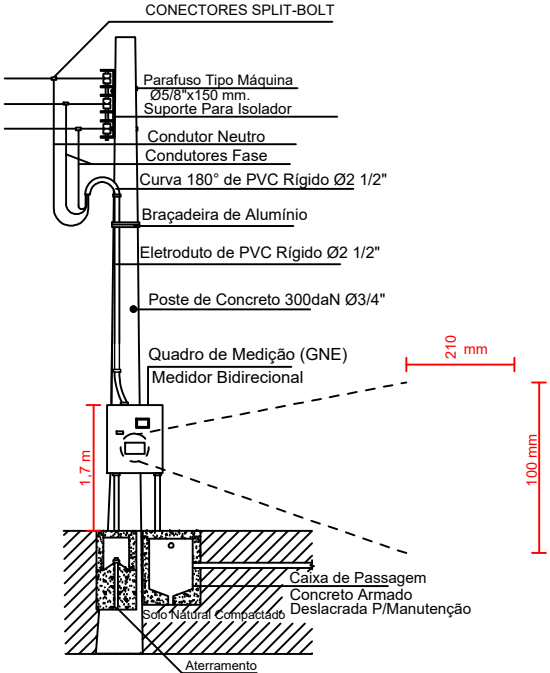
2 RAMAL DE ENTRADA E PLACA DE ADVERTÊNCIA
