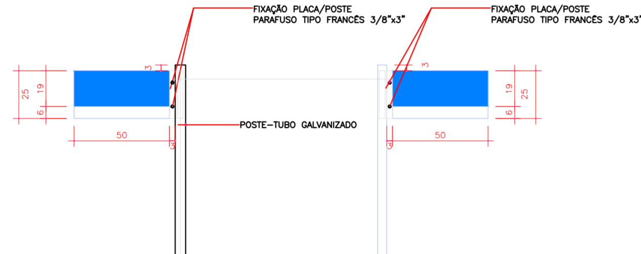
DETALHE FIXAÇÃO D1 ESCALA 1:20
