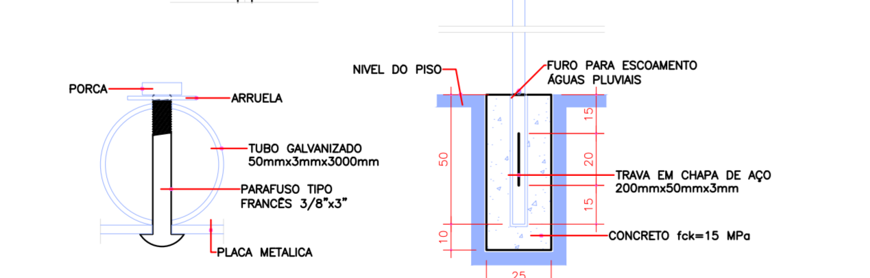
DETALHE FIXAÇÃO D1 ESCALA 1:20
