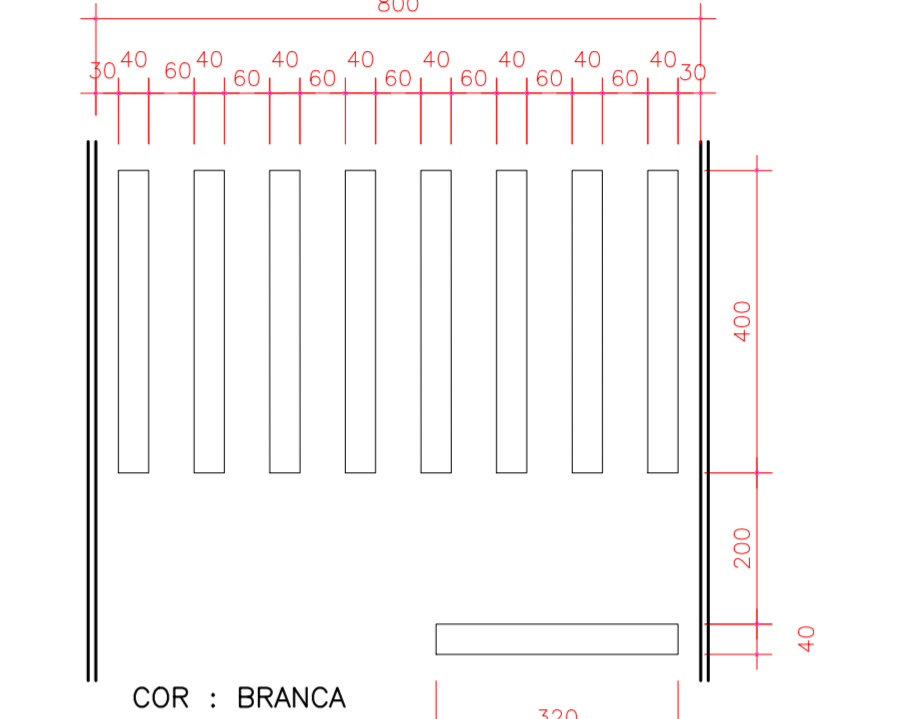
FAIXA TRAVESSIA PEDESTRES ESCALA 1:100
