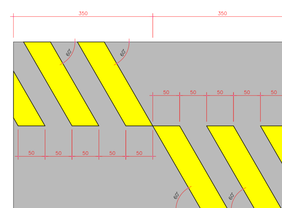
DETALHE FAIXA AMARELA LOMBADA SEM ESCALA
