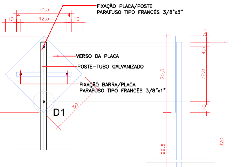
DETALHE FIXAÇÃO D1 ESCALA 1:20
