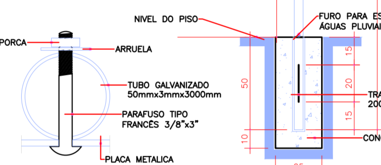
DETALHE FIXAÇÃO D1 ESCALA 1:20
