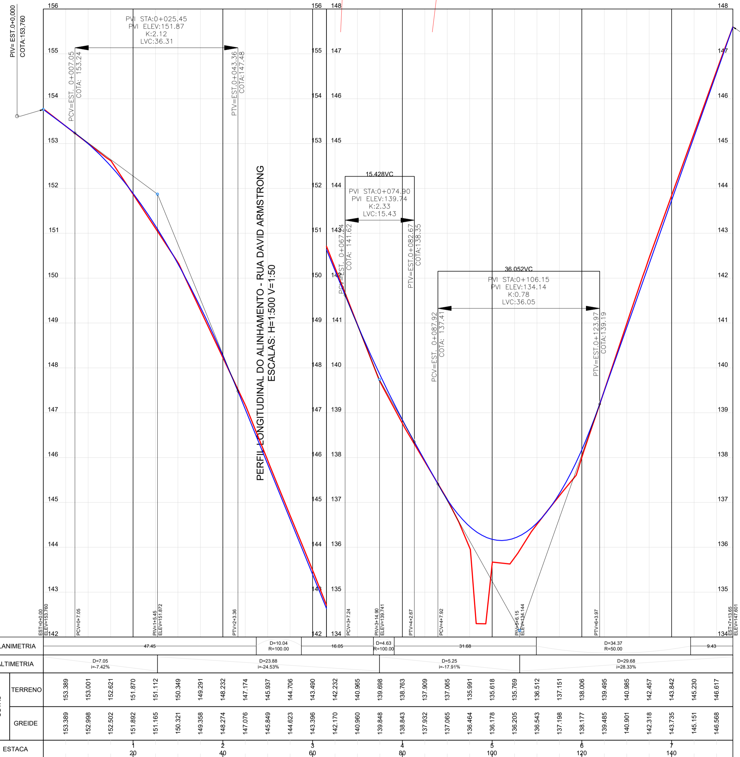
PERFIL LONGITUDINAL DO ALINHAMENTO - RUA DAVID ARMSTRONG ESCALAS: H=1:500 V=1:50
