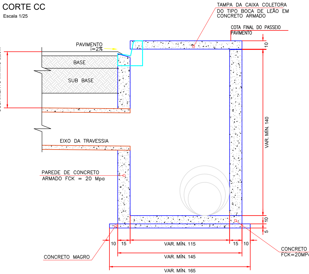
CORTE CC
