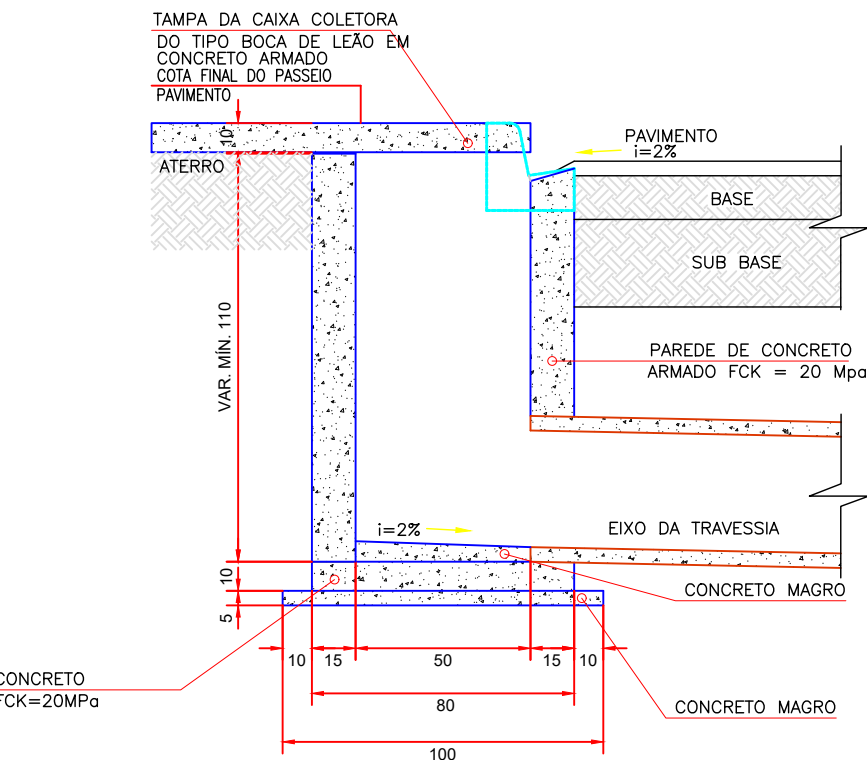
CORTE BB
