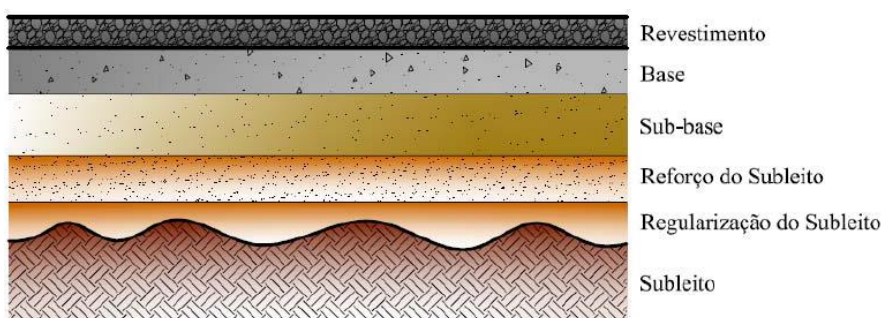
Figura 8.1 - Camadas de um pavimento flexível.
