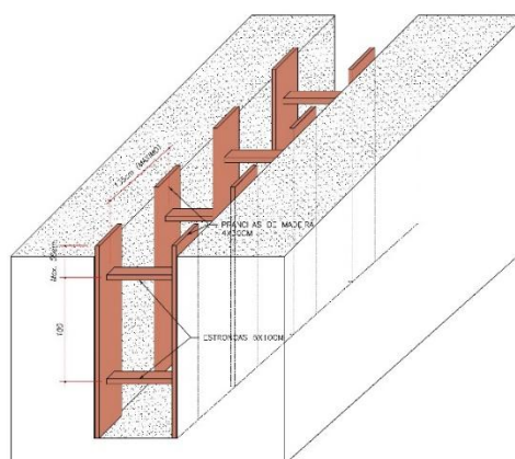
ESCORAMENTO DE VALAS TIPO PONTALETEAMENTO
