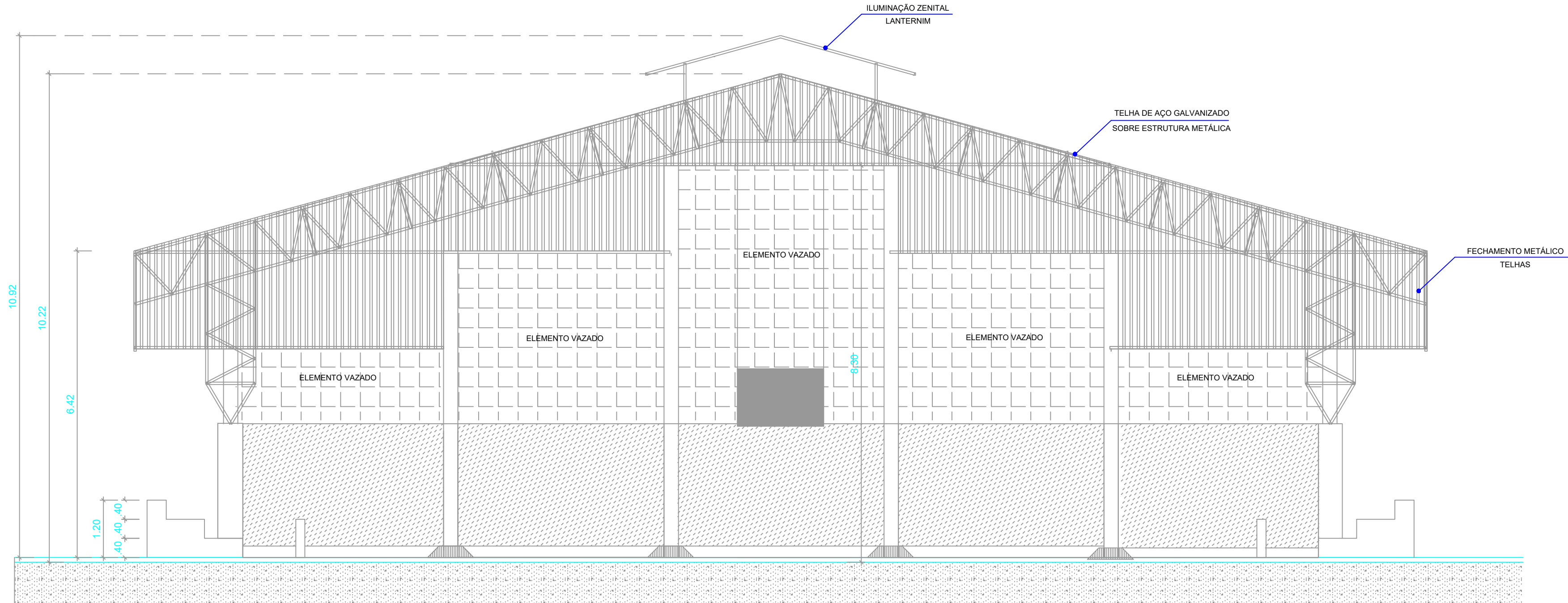
CORTE TRANSVERSAL - QUADRA POLIESPORTIVA ESC. 1/100
