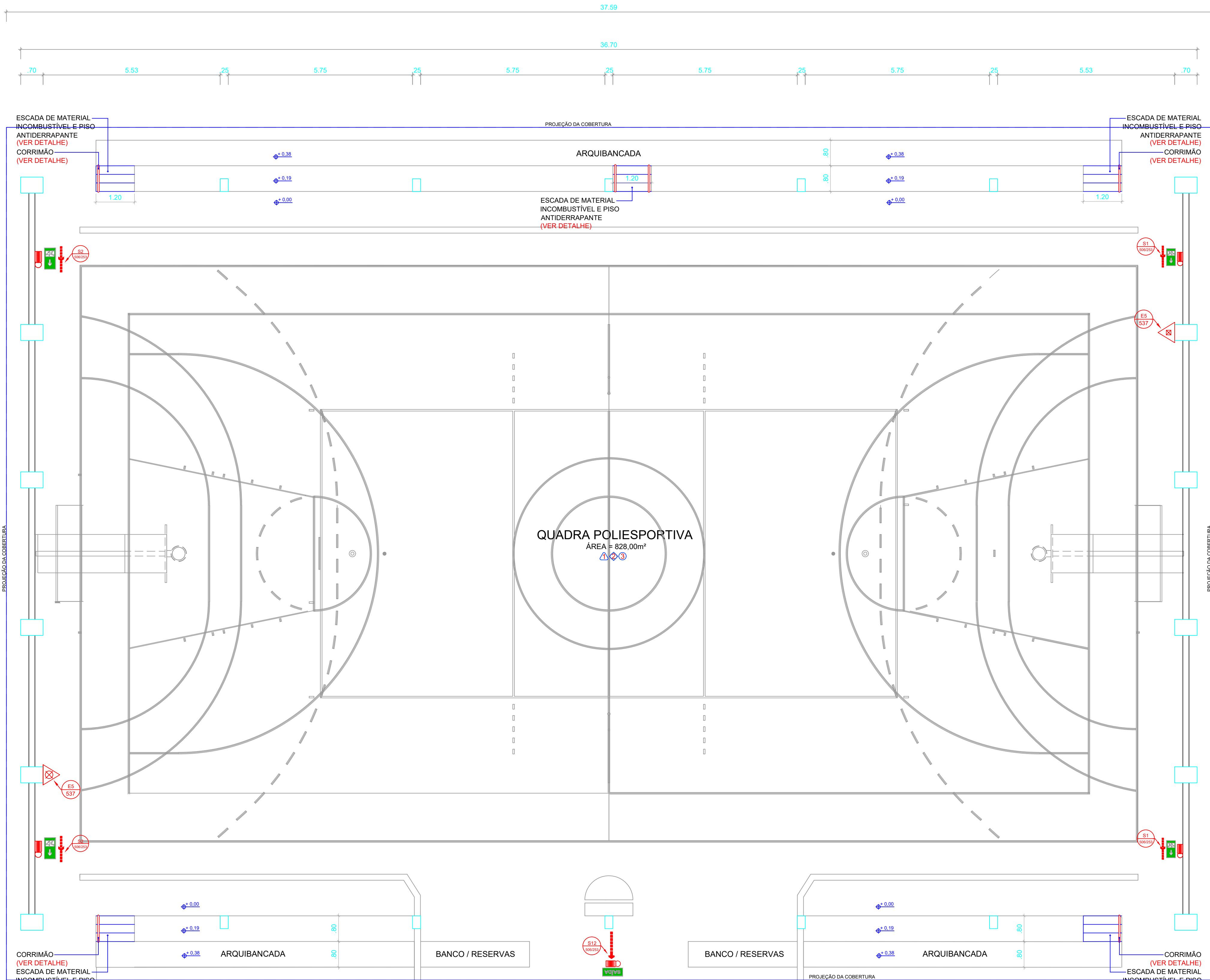
PLANTA BAIXA - BLOCO "H" / QUADRA POLIESPORTIVA ESC. 1/100 - ÁREA: 1.160,01 m²
