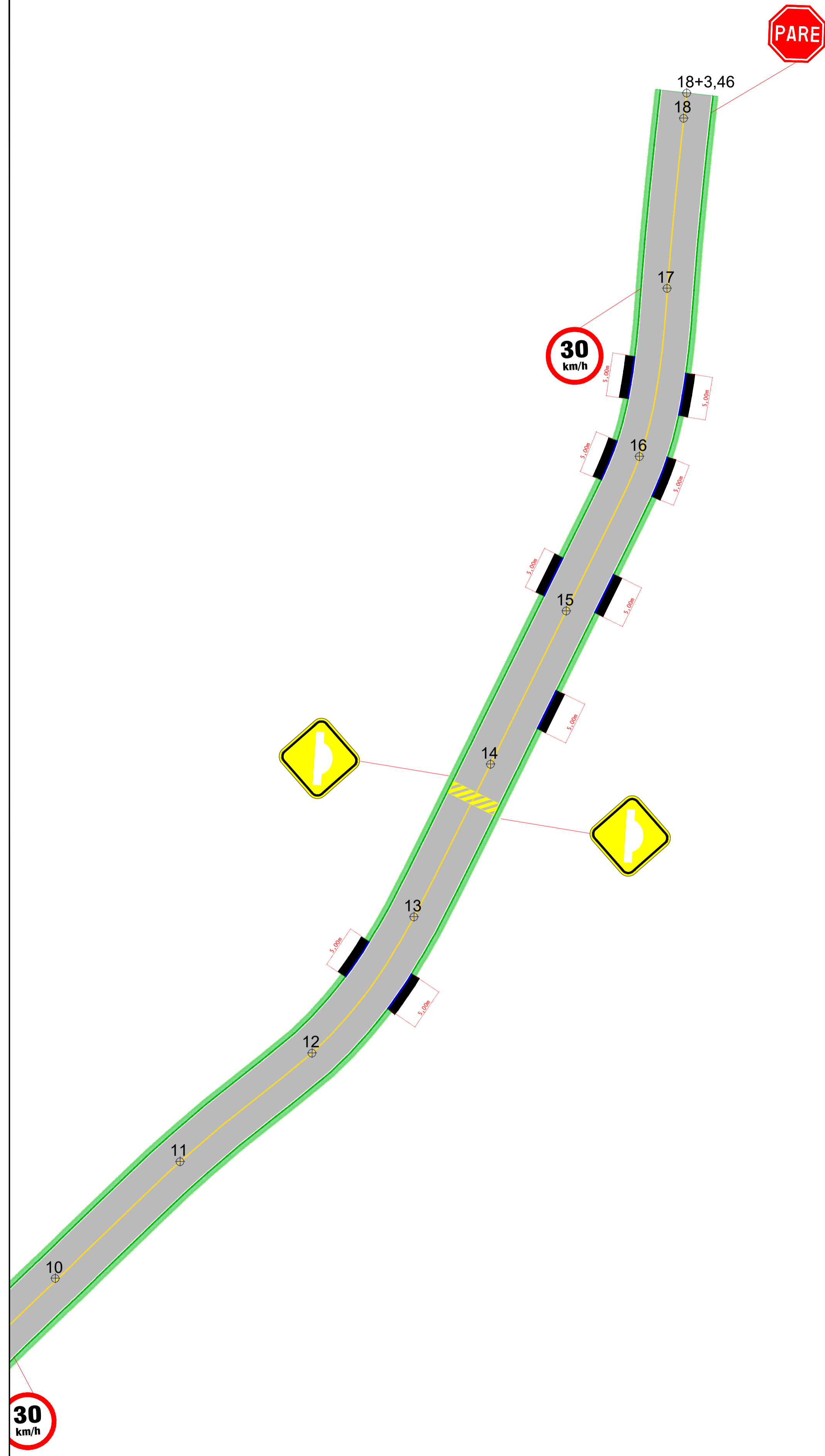
PLANTA PROJETO GEOMÉTRICO E SINALIZAÇÃO Escala: 1/300
