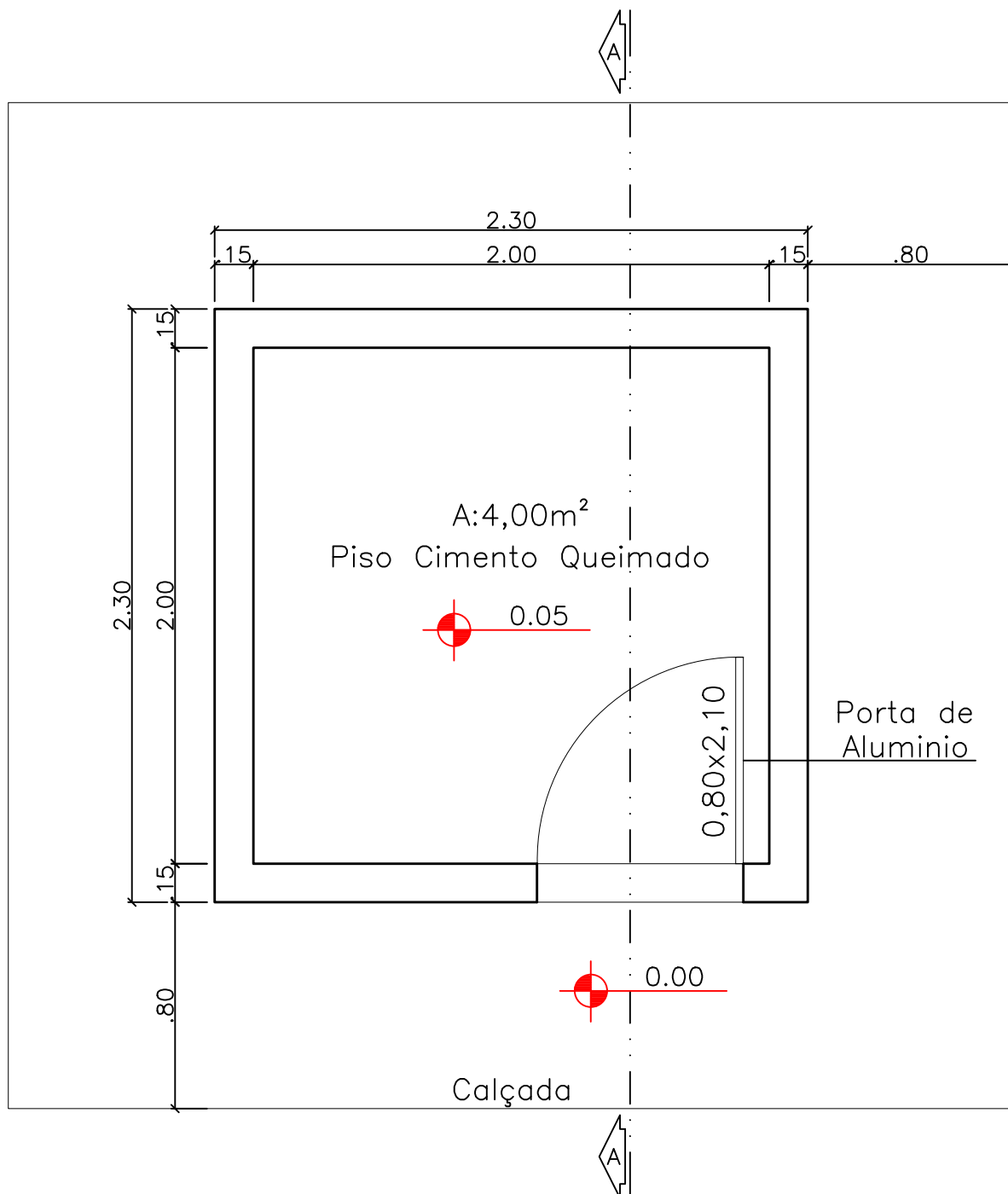
PLANTA BAIXA esc 1:25
