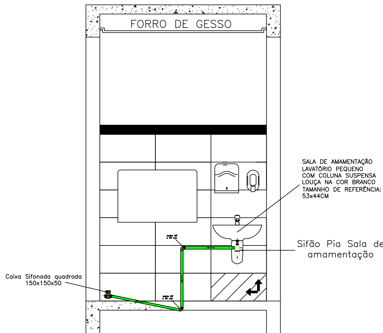
DET. SALA AMAMENTAÇÃO VISTA 01 ESCALA 1:25
