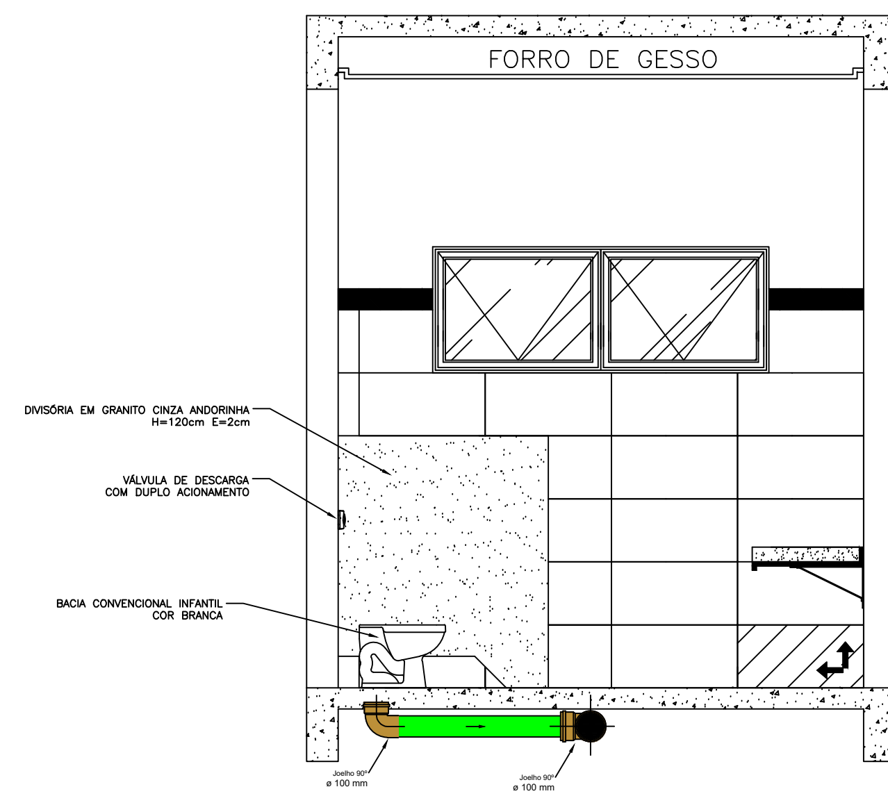
DET. I.S. INFANTIL – SALA 02 E SALA 03 VISTA 01 ESCALA 1:25
