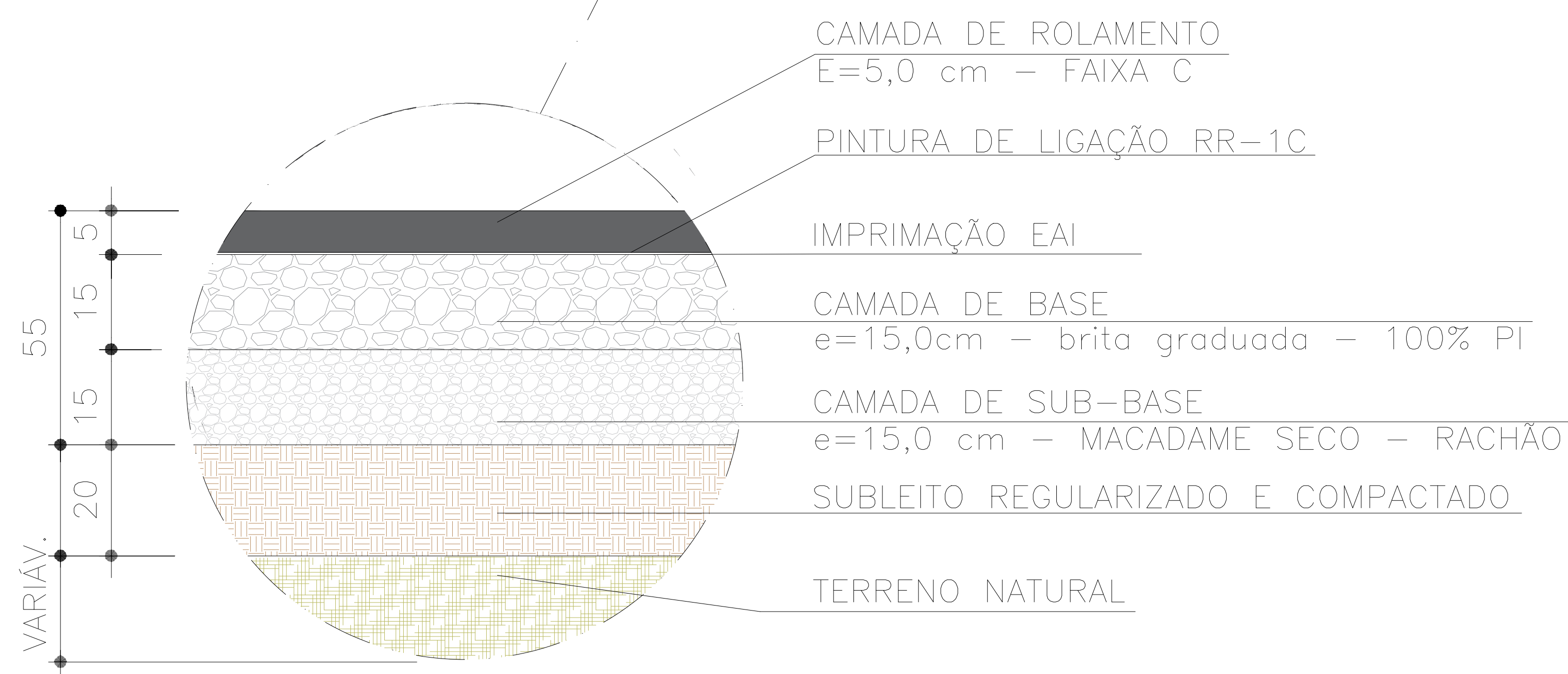
DETALHE DAS CAMADAS DE PAVIMENTAÇÃO - SOLUÇÃO 2
