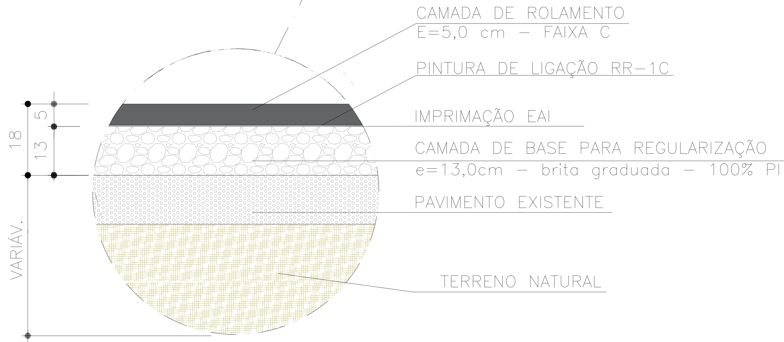
DETALHE DAS CAMADAS DE RECAPE - SOLUÇÃO 1 SEM ESCALA
