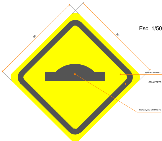
ESCALA 1/5 DETALHE A-18 | PLACA DE SINALIZAÇÃO VERTICAL OBS.: O FUNDO DAS PLACAS DEVERÃO SER EM PRETO FOSCO.
