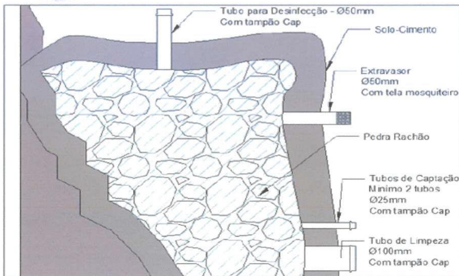
Figura com corte transversal e detalhes da tubulação necessária de nascente concluída.
