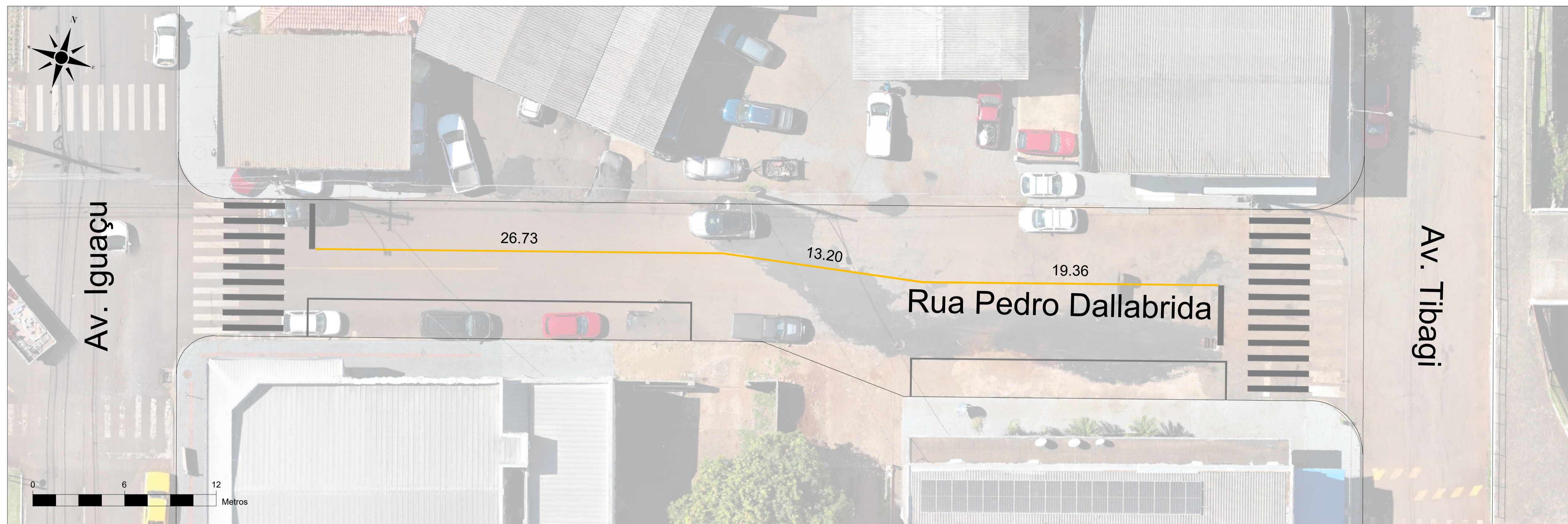
PLANTA DE SINALIZAÇÃO ESCALA: 1/150
