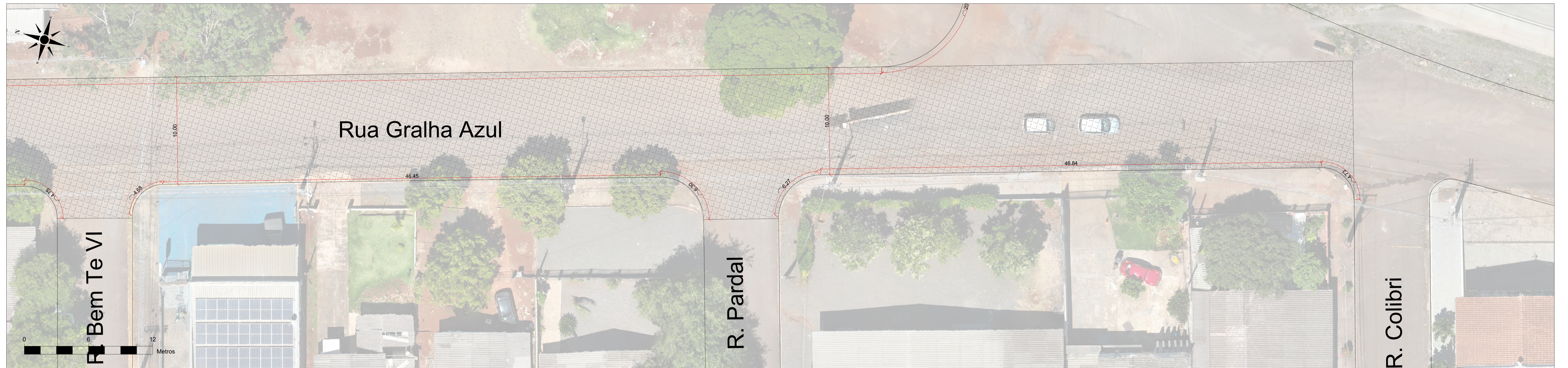
PLANTA GEOMÉTRICA E PAVIMENTAÇÃO ESCALA: 1/150
