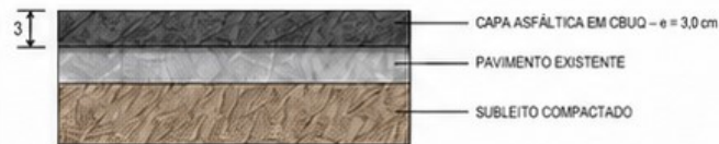
DETALHE TÍPICO 02 – RECAPE ASFÁLTICO SEM ESCALA
