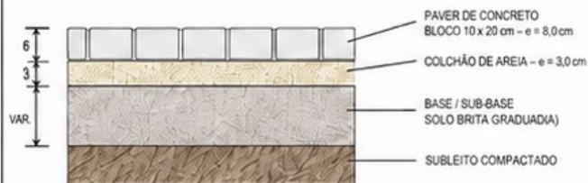
DETALHE TÍPICO 01 – PAVIMENTO INTERTRAVADO SEM ESCALA
