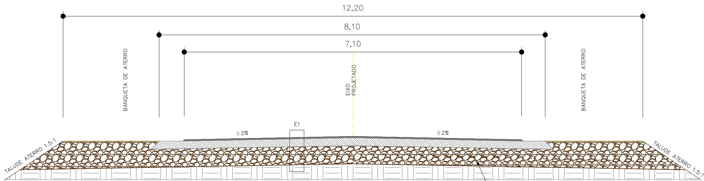
DETALHE SEÇÃO TIPO – 01 – (PARA TRECHO COM ELEVÇÃO DO GREIDE E READEQUAÇÃO DA ESTRADA) SEM ESCALA
