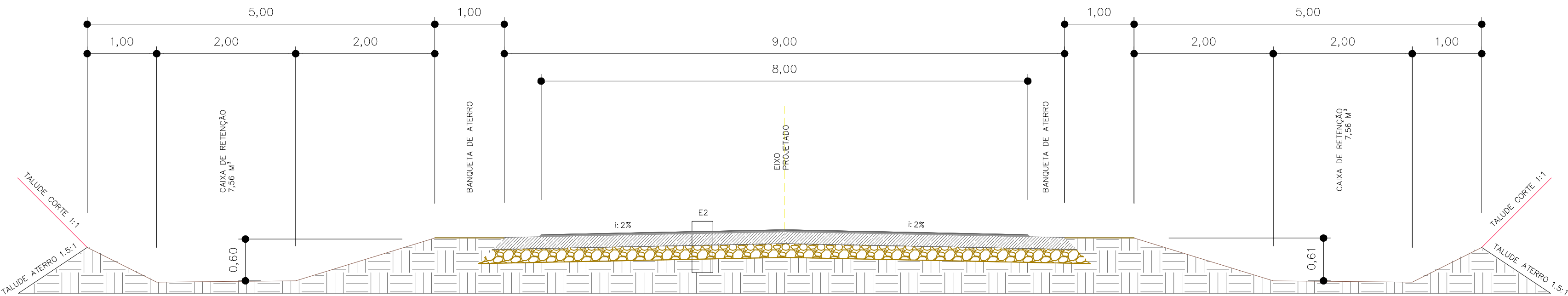
DETALHE SEÇÃO TIPO – 03 (PARA TRECHO COM CAIXA DE RETENÇÃO) SEM ESCALA
