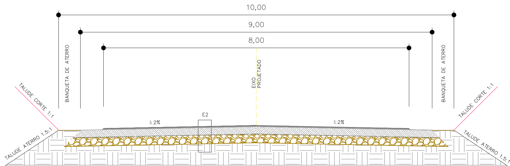
DETALHE SEÇÃO TIPO – 02 SEM ESCALA
