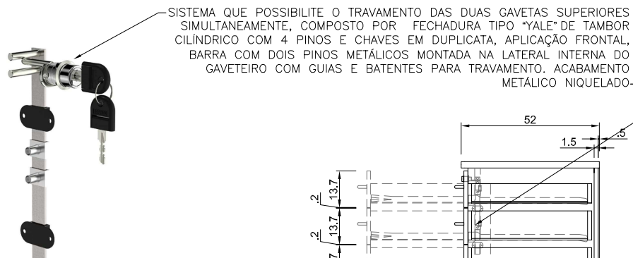
SEÇÃO 3 ESC.:1/20
