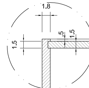
DETALHE "A" ESC.:1/5
