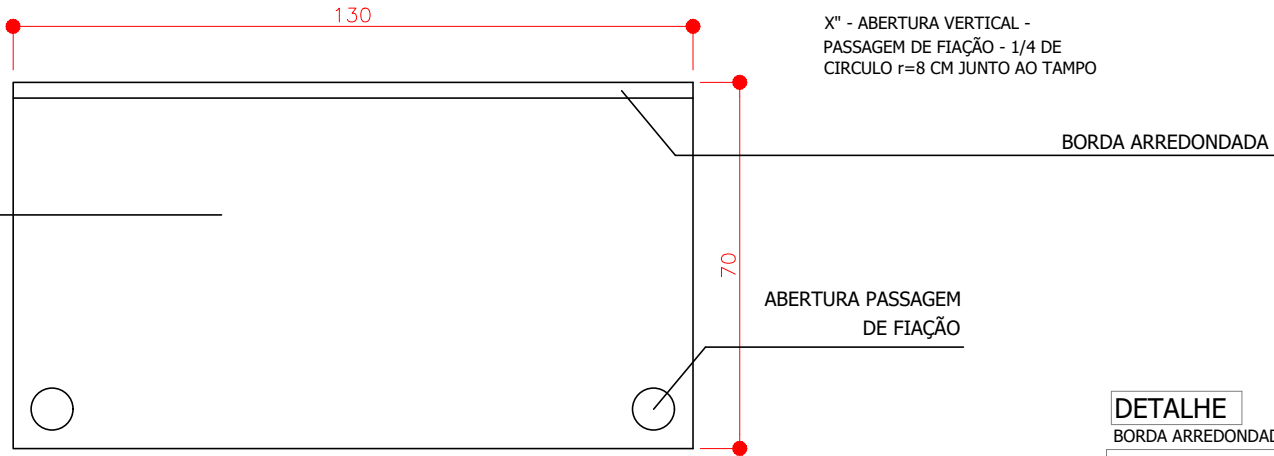
PLANTA DE TOPO
