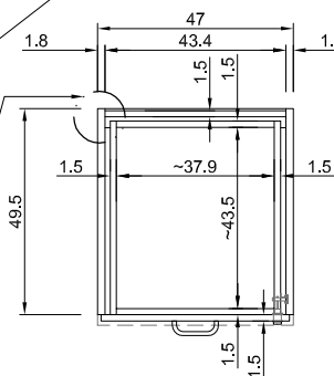
SEÇÃO 1 ESC.:1/20
