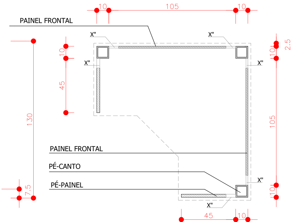
PLANTA DE CORTE
