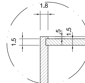
DETALHE "A" ESC.:1/5
