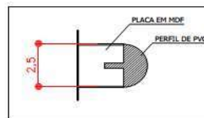
DETALHE: ENCABEÇAMENTO DA BORDA
