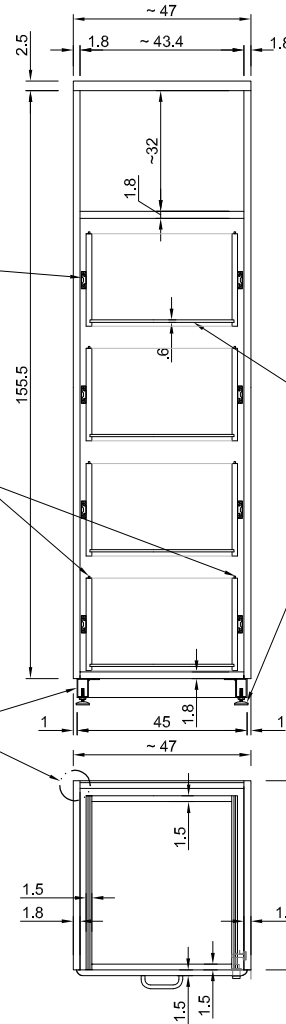
SEÇÃO 2 ESC.:1/20
