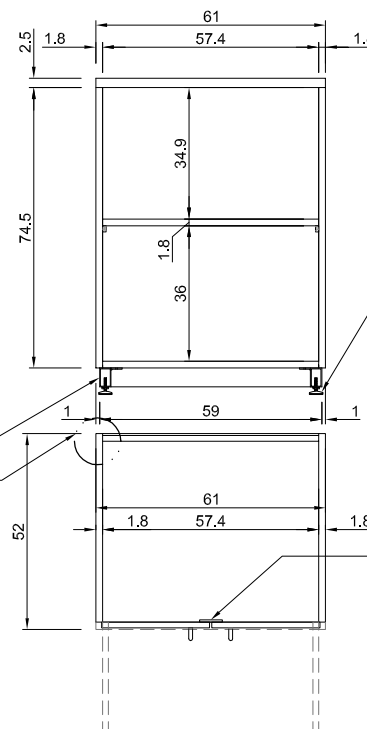
SEÇÃO 2 ESC.:1/20
