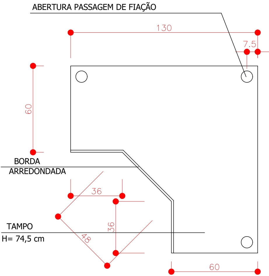
PLANTA DE TOPO
