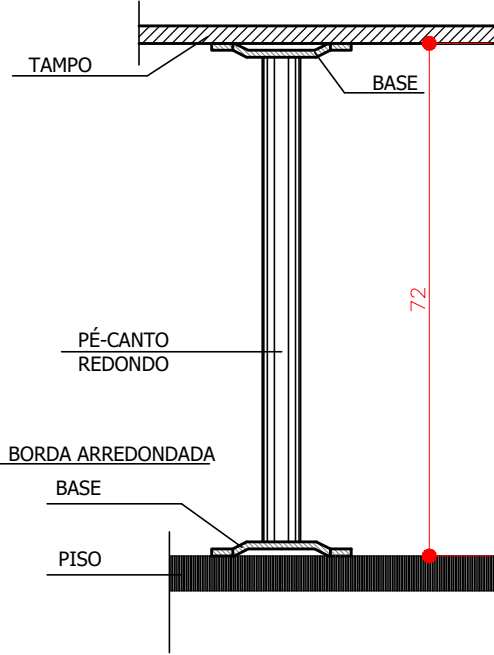
DETALHE CORTE - PÉ-CANTO REDONDO
