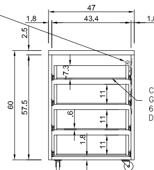
SEÇÃO 2 ESC.:1/20
