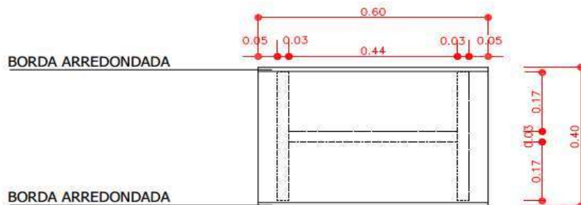
PLANTA DE TOPO
