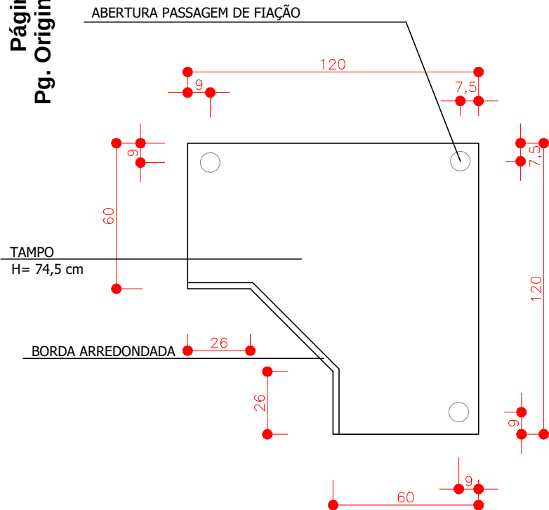
PLANTA DE TOPO
