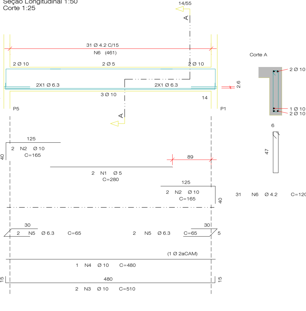
V12 Seção Longitudinal 1:50 Corte 1:25
