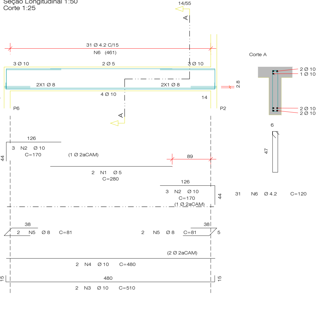
V16 Seção Longitudinal 1:50 Corte 1:25
