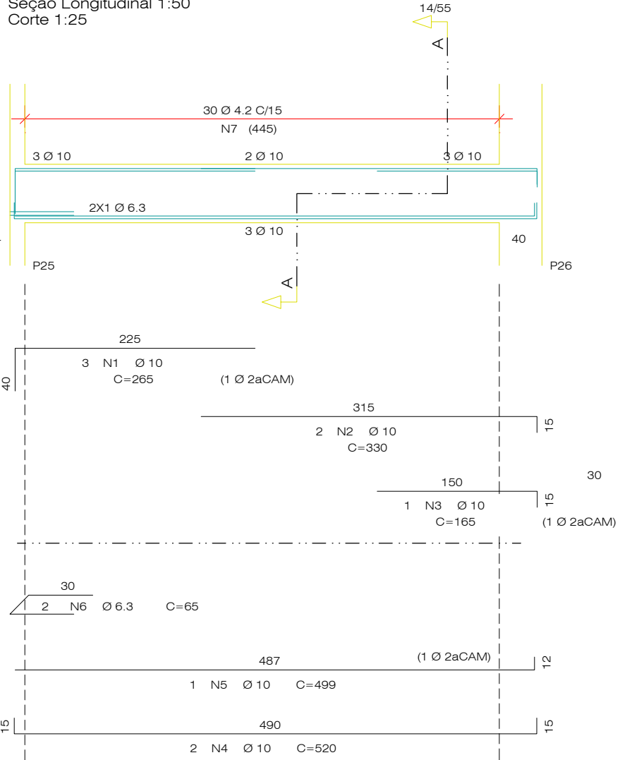
V9 Seção Longitudinal 1:50 Corte 1:25
