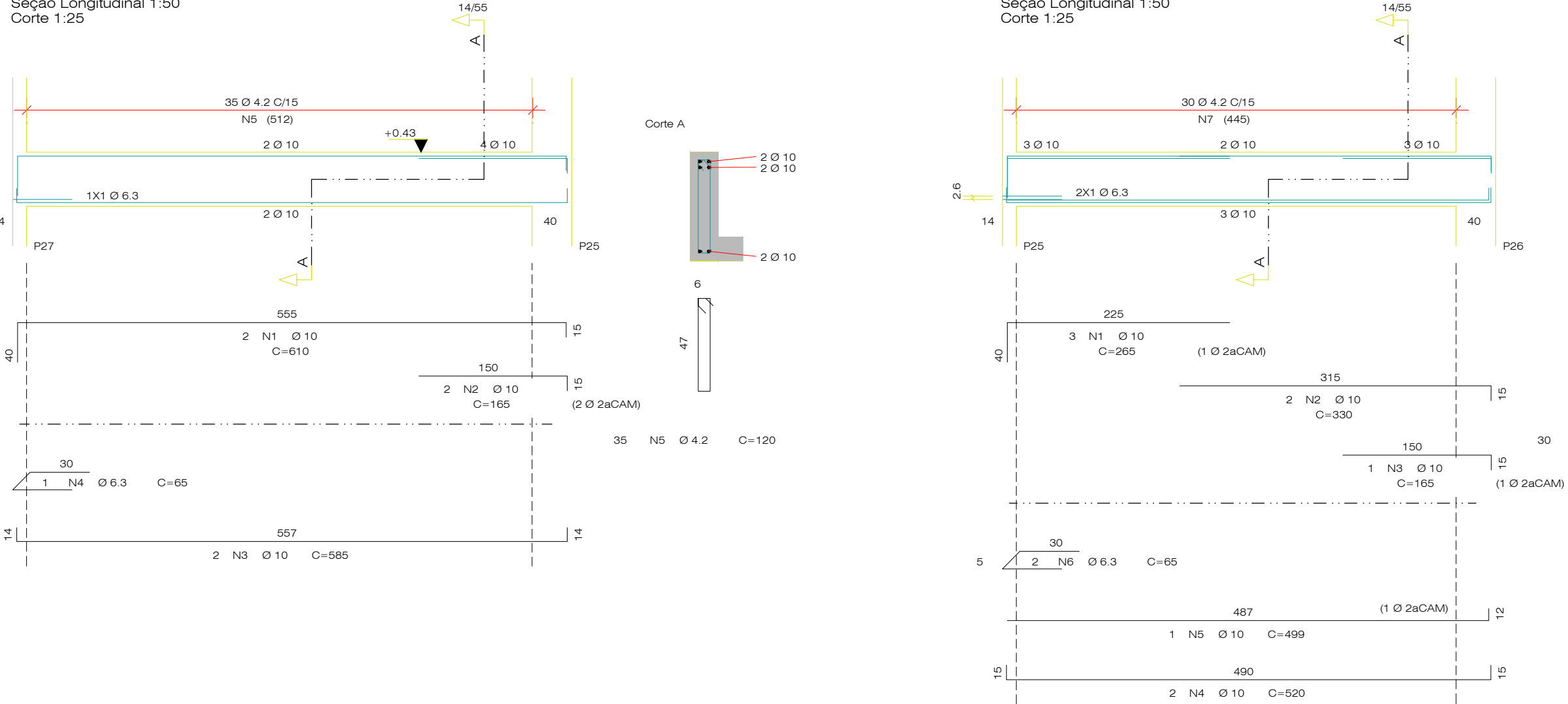
V10 Seção Longitudinal 1:50 Corte 1:25
