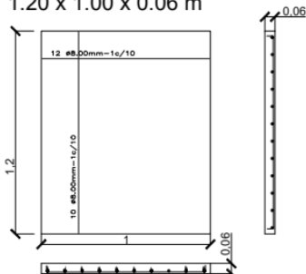
Armadura Boca de Lobo 1.20 x 1.00 x 0.06 m
