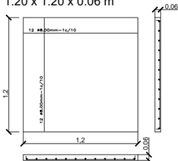
Armadura Boca de Lobo 1.20 x 1.20 x 0.06 m
