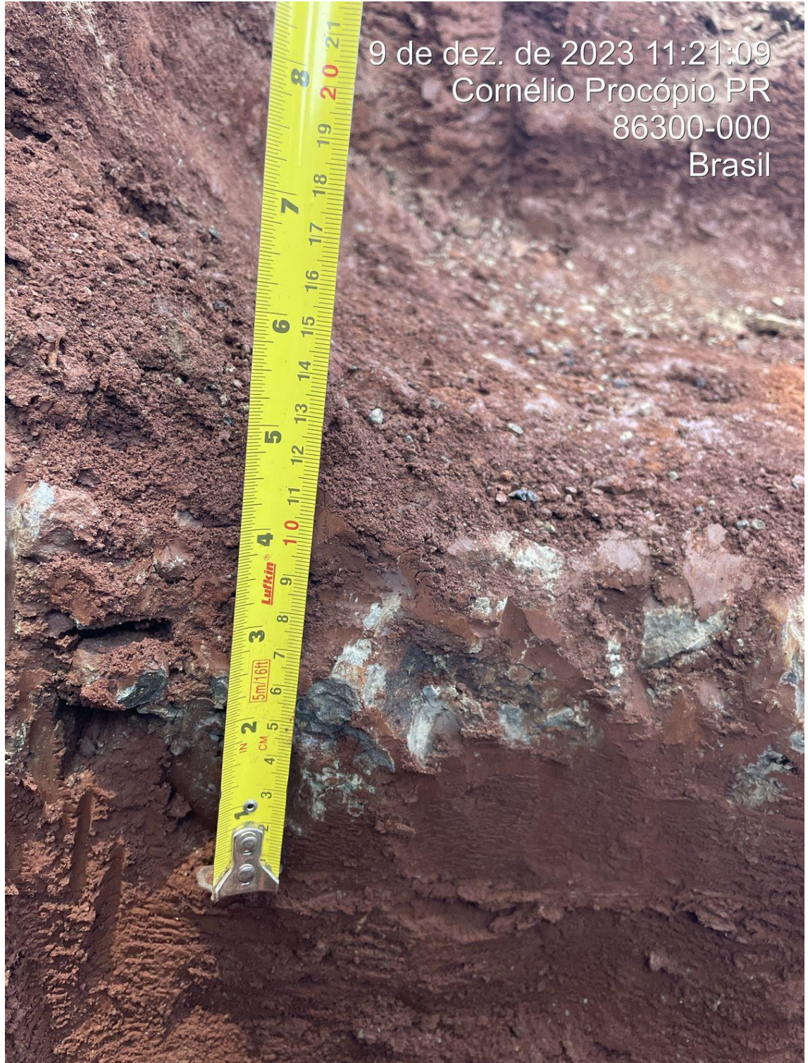
Figura 7. Medição da espessura da sub-base. Fonte: os Autores.
