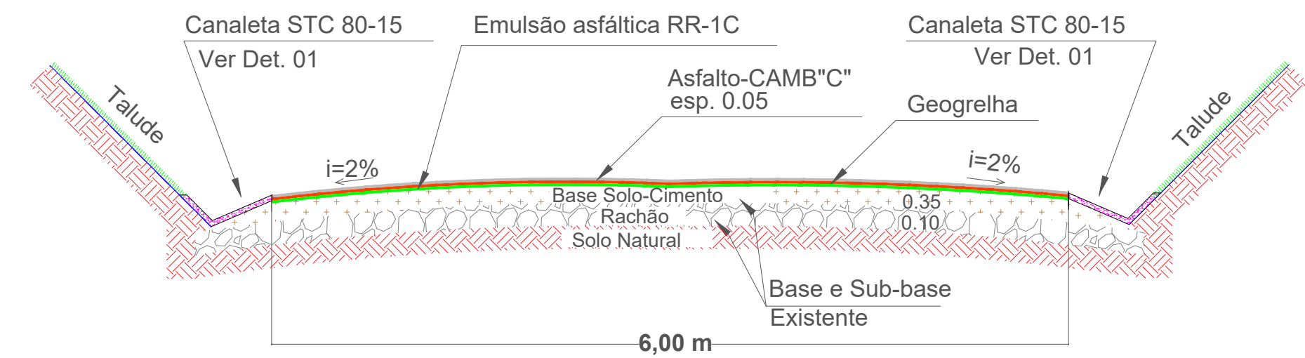
DETALHE Corte Seção Esquemático Estacas: 0PP á 125 S/ESC
