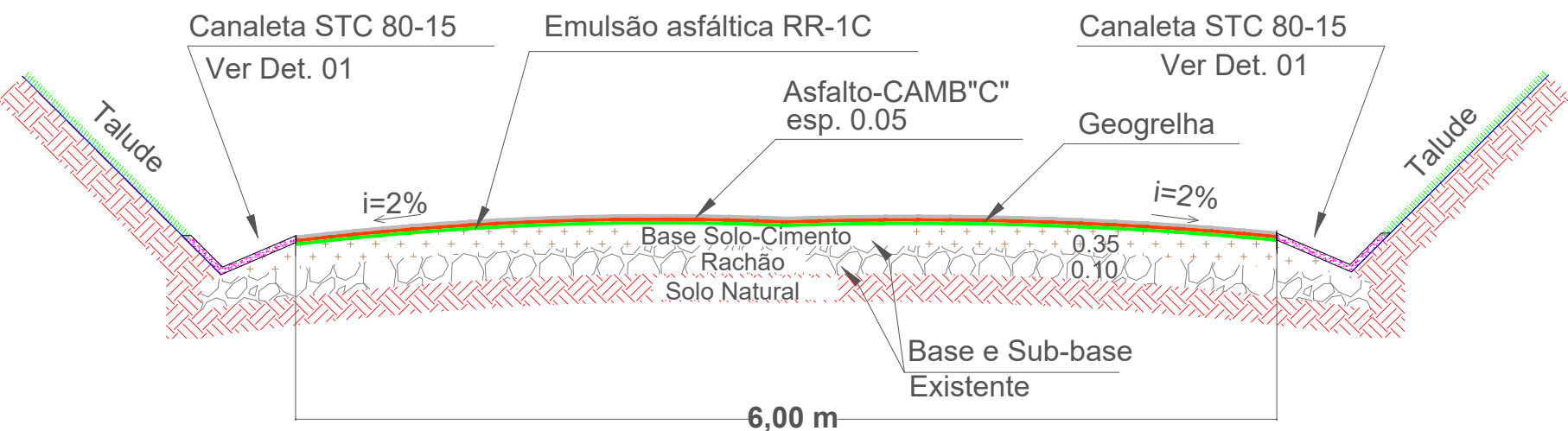
DETALHE Corte Seção Esquemático
