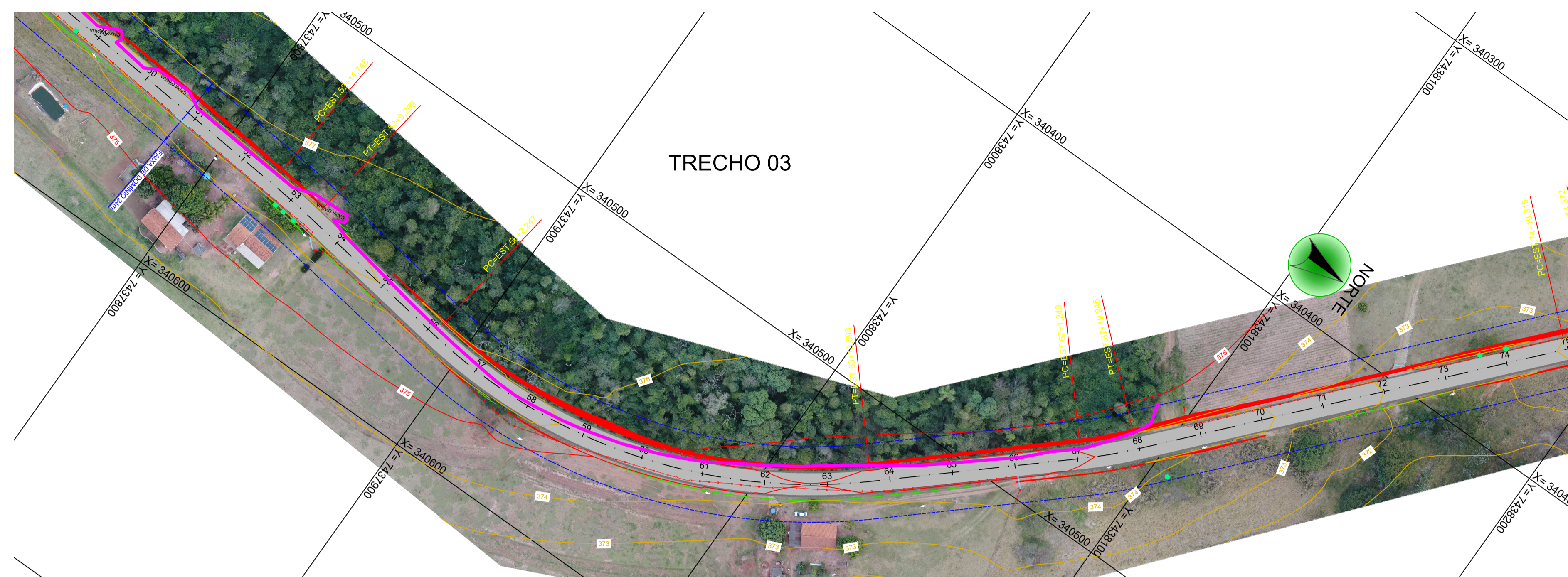
PLANTA BAIXA - EXECUTIVO ESC. 1/1000
