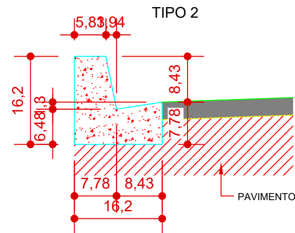
Detalhe do Meio-fio ESCALA: 1:25
