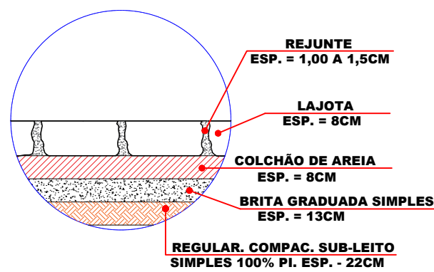
Seção Transversal SEM ESCALA
