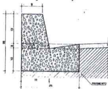
Figura 4 – Representação Meio-fioTipo2 DER/PR
