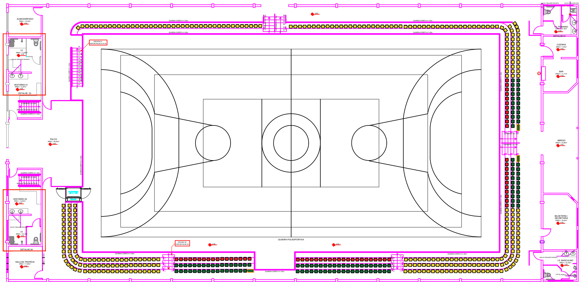
PLANTA BAIXA CADEIRAS ESCALA 1:75
