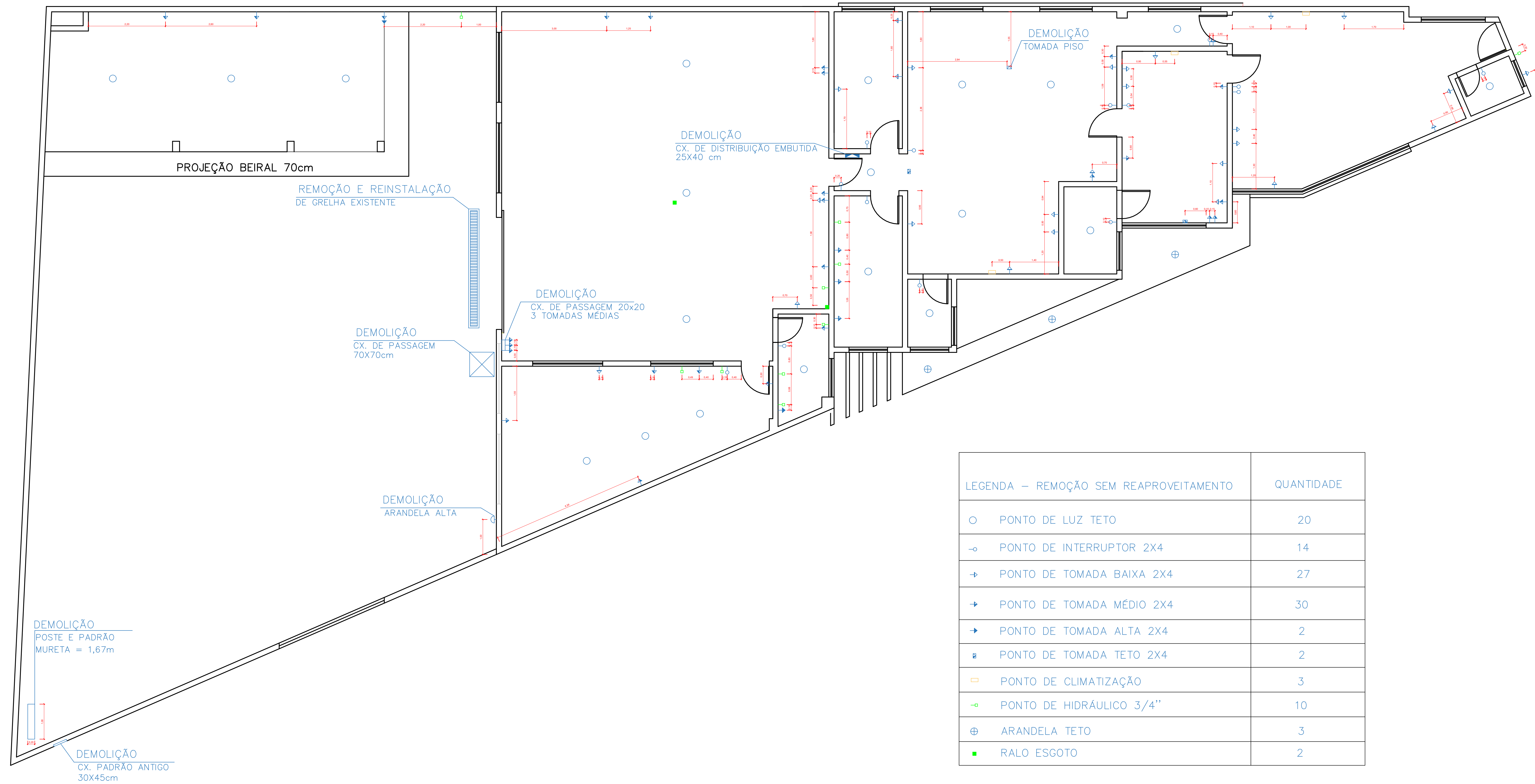
1 PLANTA BAIXA - DEMOLIÇÃO PONTOS ELÉTRICOS E HIDRÁULICOS ESCALA 1/50
