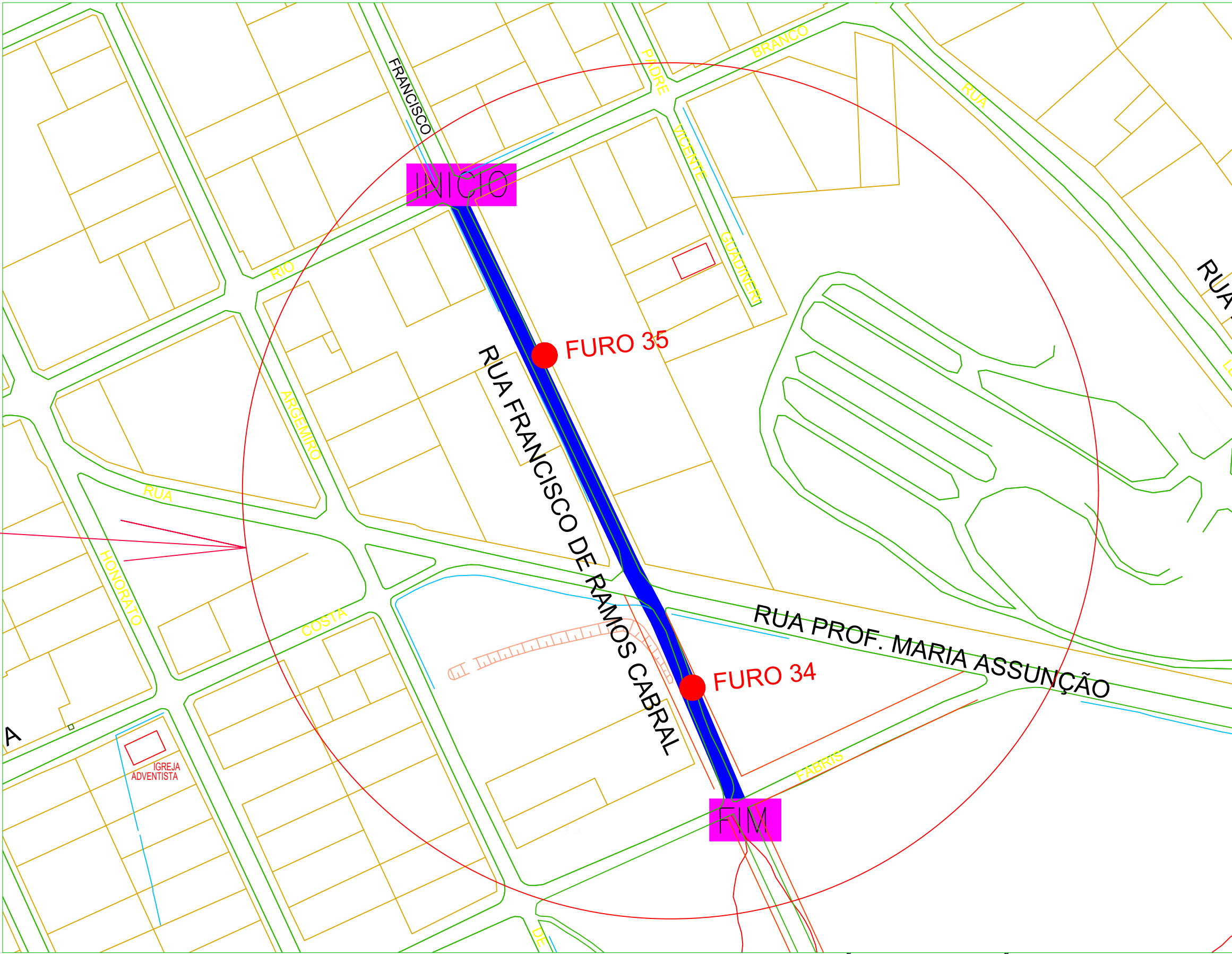
PLANTA DE IMPLANTAÇÃO DA PAVIMENTAÇÃO
